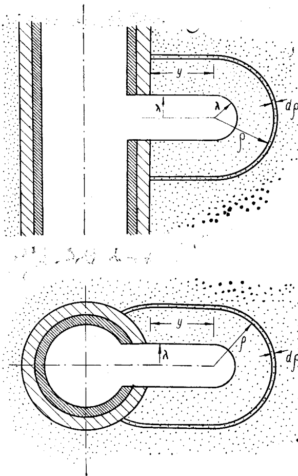
Рис. 1. Схема отверстия в колонне и цементном кольце скважины с каналом радиуса \lambda и длиной цилиндрической части y и выделенного вокруг него тонкостенного тела, нужного для вывода формулы геометрической характеристики зоны влияния этого канала. Вверху продольный разрез, внизу поперечный. Плотной косоштриховкой заштрихована обсадная колонна, редкой штриховкой—цементное кольцо
