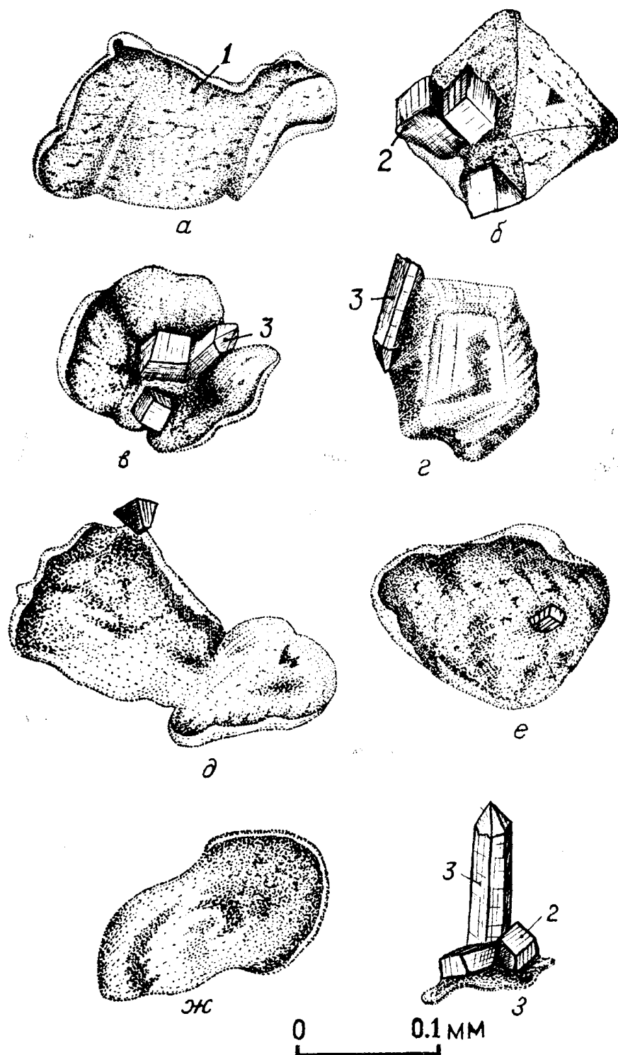
Рис. 1. Морфология золотины из россыпей района г. Томска: а, д, е, ж — лепестковидная форма золотины с загнутыми краями; б — толстотаблитчатая золотины в сростании с окисленным пиритом (2); в, з — лепестковидные золотины в сростании с пиритом (2) и кварцем (3); г — толстотаблитчатая золотины в сростании с кварцем (3)
