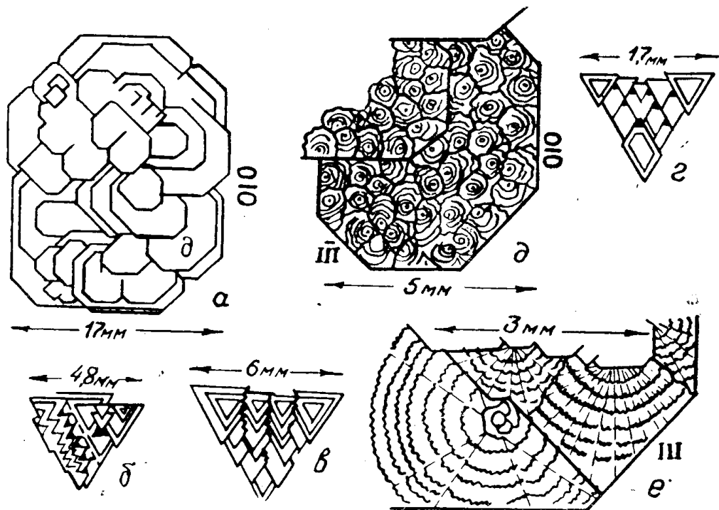
Рис. 5. Блоковое строение кристаллов пирита. a — пластинчатые блоки пирита, слагающие грань куба; b, v, z — блоковое строение граней октаэдра; d — деталь строения поверхности одного из блоков, на которой ясно заметны концентрические слои роста. e — деталь, поясняющая характер строения концентрических слоев роста поверхности куба
