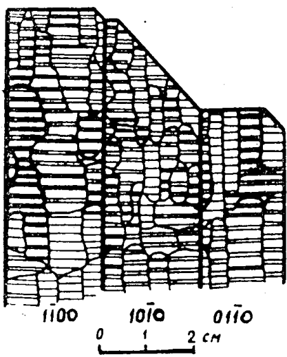
Рис. 10. Блоковое строение граней (1100) , (1010) и (0110) кристалла горного хрусталя.
