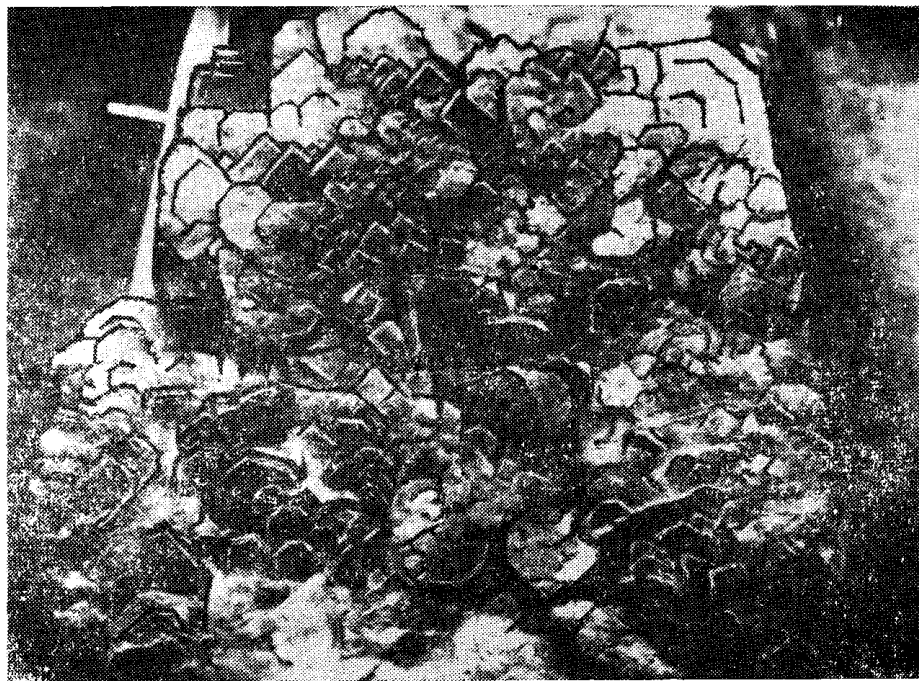
Рис. 1. Поверхность куба кристалла галенита, сложенная кристаллитами нескольких порядков
