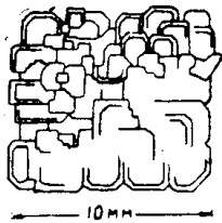
Рис. 3. Зарисовка поверхности куба флюорита, сложенной пластинчатыми кристаллитами нескольких порядков (а); б — деталь строения одного из участков описываемого флюорита
