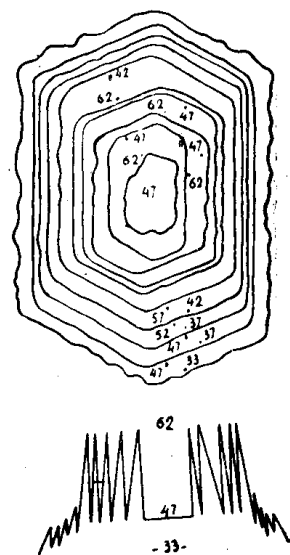
Рис. 17. Зонарный плагиоклаз
