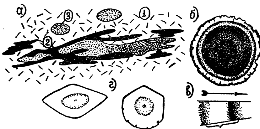
Рис. 1. Выделения гиббсита и морфология оолитов в осадке. а) полости, выполненные гиббситом: 1—основная масса породы, 2—лимонит, 3—гиббсит. Увел. 15 x ; б) увеличение содержания гидрата окиси железа (темное) к центру оолитовой постройки. Увел. 300 x ; в) асимметричное распределение гидрата окиси железа в концентриках (стрелкой указано направление диффузии внешнего компонента); г) выделения гиббсита в глинистой массе породы. Увел. 900 x ;
