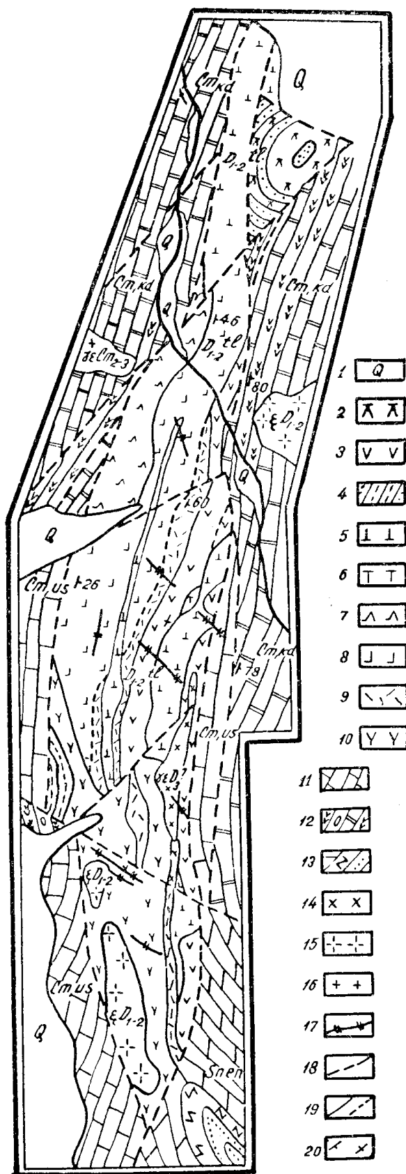
Рис. 1. Схематическая геологическая карта Талановского грабена (составили В. Г. Крюков, Н. С. Лыхина, В. З. Мустафин): 1—аллювиальные отложения. Среднедевонские: 2—андезитовые порфириды; 3—базальтовые, оливинпироксеновые порфириды и кластолавы; 4—красноцветные и сероцветные конгломераты, песчаники, алевролиты. Нижнедевонские: 5—рахитовые порфиры, ортофиры; 6—трахандезитовые порфириды; 7—роговообманковые порфириды; 8—лабрадорпироксеновые и лабрадоровые порфириды; 9—лавы и кластолавы лабрадорпироксеновых порфиритов; 10—нерасчлененные порфириды основного состава; 11—известняки, сланцы и эффузивы усинской свиты; 12—порфириды, порфиритоидные альбитофиры, сланцы, известняки и силицилитовые конгломераты кондомской свиты; 13—битуминозные известняки, кремнистые сланцы, силицилиты енисейской свиты. Девонские интрузии: 14—граносиениты; 15—сиениты, щелочные сиениты; 16—гранодиориты и плагиограниты мартайгинского комплекса; 17—дайки; 18—дизъюнктивы; 19—геологические границы: литологические и фациальные; 20—элементы залегания.
