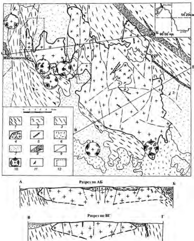
Рис. 1. Структурно-тектоническая схема НКМ: 1 – гнейсовый комплекс (AR); 2 – приконтактовая мигматизация; 3 – слюдяно-гнейсовый комплекс с амфиболитами, кварцитами и мраморами (AR – PR); 4 – контур гранитоидов НКМ: а – диориты и гранодиориты 1-й фазы, б – граниты и лейкограниты 2-й фазы; 5 – дайки кислого состава; 6 – терригенно-вулканогенные отложения (PZ2); 7 – терригенные отложения (J); 8 – зоны мylonитов; 9 – основные разломы, выделенные по геолого-геофизическим и структурно-геоморфологическим данным; 10 – круговые диаграммы ориентировки трещин; 11 – элементы залегания пород; 12 – контуры участков детальных исследований (с юго-востока на северо-запад – «Каменный», «Итатский», «Енисейский»)
