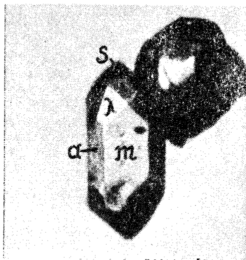
Рис. 2. Кристалл акцессорного циркона 8 типа. Увеличение 250\times . a\{100\} , m\{110\} , \lambda\{311\} , S\{111\} .
