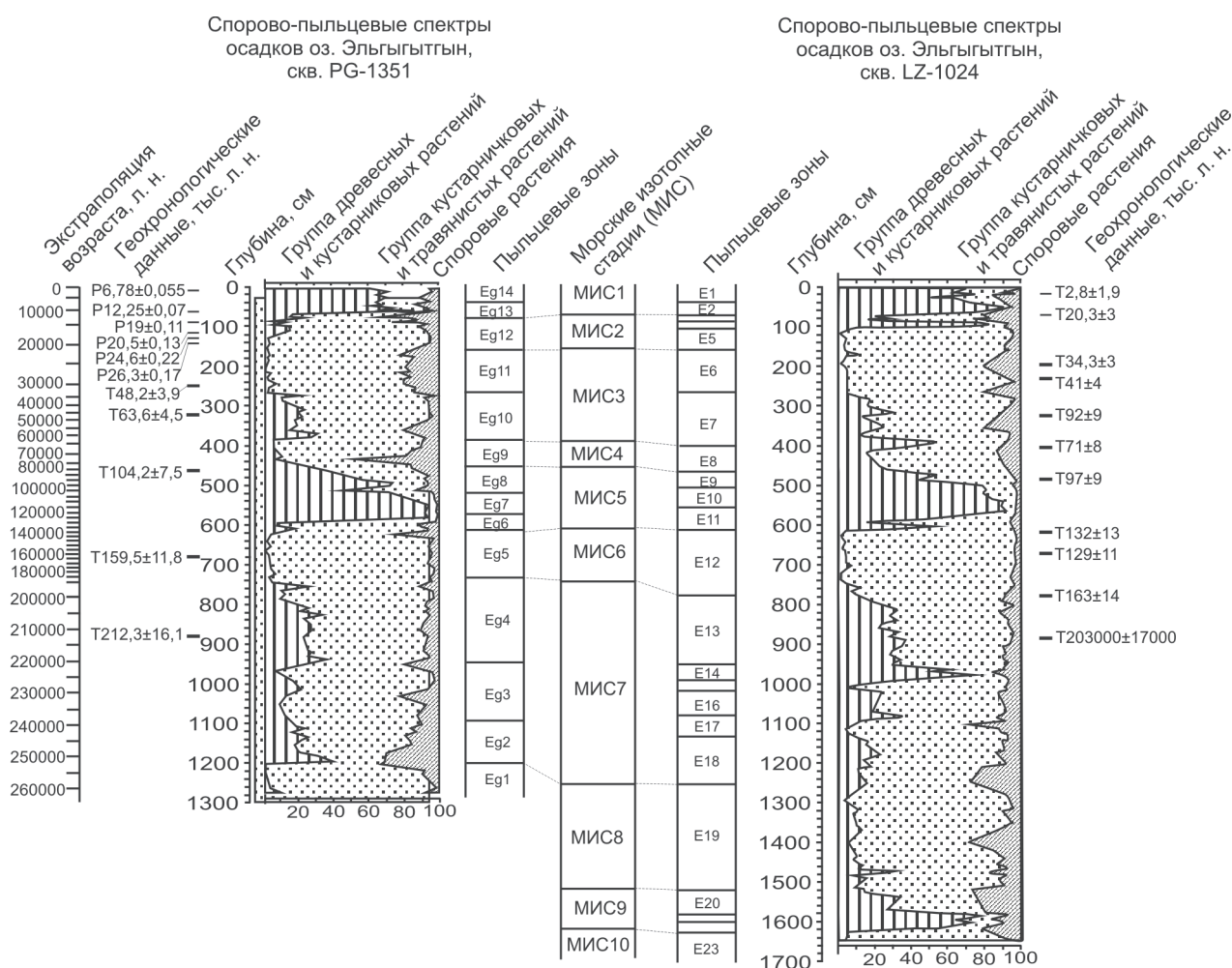
Рис. 3. Корреляция пыльцевых зон кернов скв. PG-1351 и LZ-1024 осадков оз. Эльгыгытгын с морскими изотопными стадиями: P – радиоуглеродные данные (Forman et al., 2007), T – термолюминесцентные (Juschus et al., 2007)
