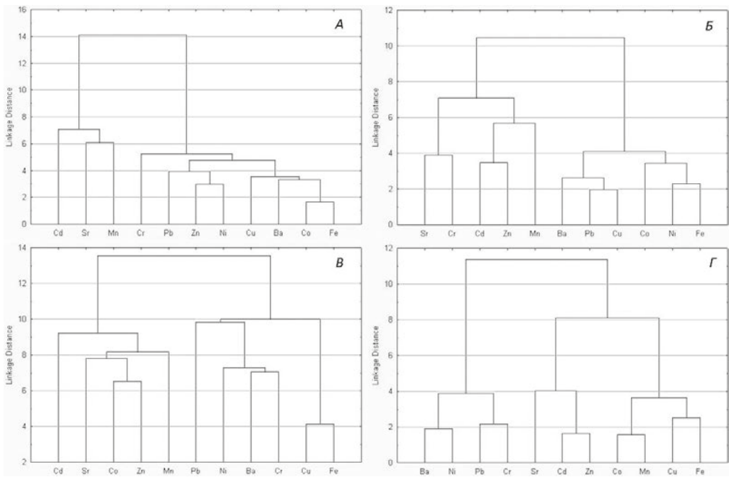
Рис. 1. Дендрограммы кластерного анализа нормализованных данных по содержанию МЭ для: а — листьев липы, б — листьев тополя, в — корки липы, г — корки тополя.
