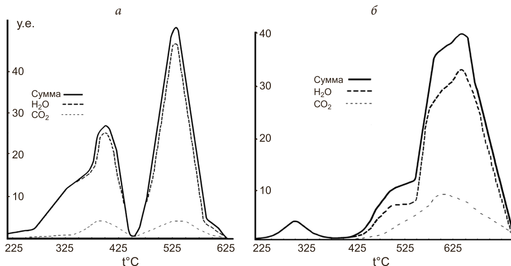
Рис. 8. Графики зависимости состава и выхода массовой доли газовой-жидкой фазы ( H_2O , CO_2 и их суммарной массы, в условных единицах — у.е.) от температуры декрипитации флюидных включений в порфировидном кварце из пород Салминского массива: а — кварц из гранитов рапакиви, б — ксеногенный кварц из гибридной базальтовой дайки
