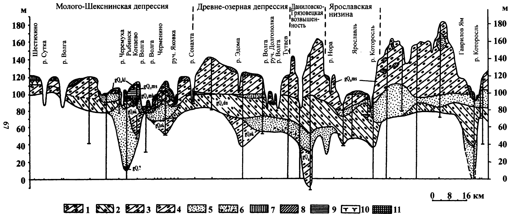
Рис. 1. Схематический геологический разрез плейстоценовых отложений Ярославского Поволжья (по Судаковой Н. Г. [Проблемы..., 2001а]) 1–4 – моренные горизонты: 1 – окский, 2 – днепровский, 3 – московский, 4 – подпорожский (бывший калининский); 5 – песок; 6 – песок с галькой; 7 – покровные лессовидные отложения; 8 – суглинок; 9 – глина; 10 – псевдоморфозы по морозобойным клиньям; 11 – гиттия
