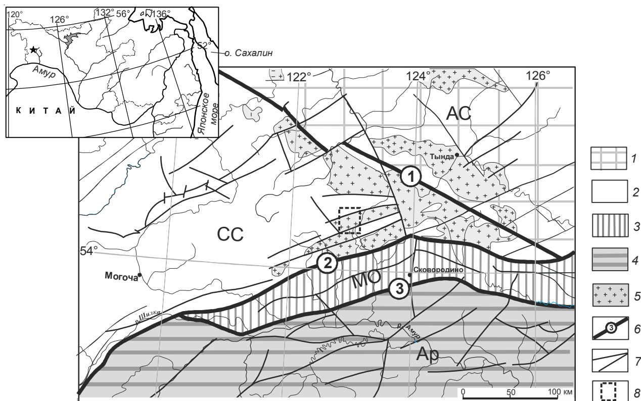
Рис. 1. Схема распространения интрузивных массивов позднепалеозойского и тукурингского комплексов в пределах юго-восточного обрамления Северо-Азиатского кратона. Составлена авторами по материалам [6, 7, 9, 33]. 1 – Алдано-Становой щит (АС); 2–4 – орогенные пояса: 2 – Селенгино-Становой (СС), 3 – Монголо-Охотский (МО), 4 – Аргунский (Ар); 5 – гранитоиды позднепалеозойского и тукурингского комплексов; 6 – основные региональные разломы (1 – Желтулакский, 2 – Северо-Тукурингский, 3 – Южно-Тукурингский); 7 – тектонические нарушения; 8 – район расположения Хайктинско-Орогжанского массива. На врезке звездочкой показано географическое положение Березитового месторождения.
