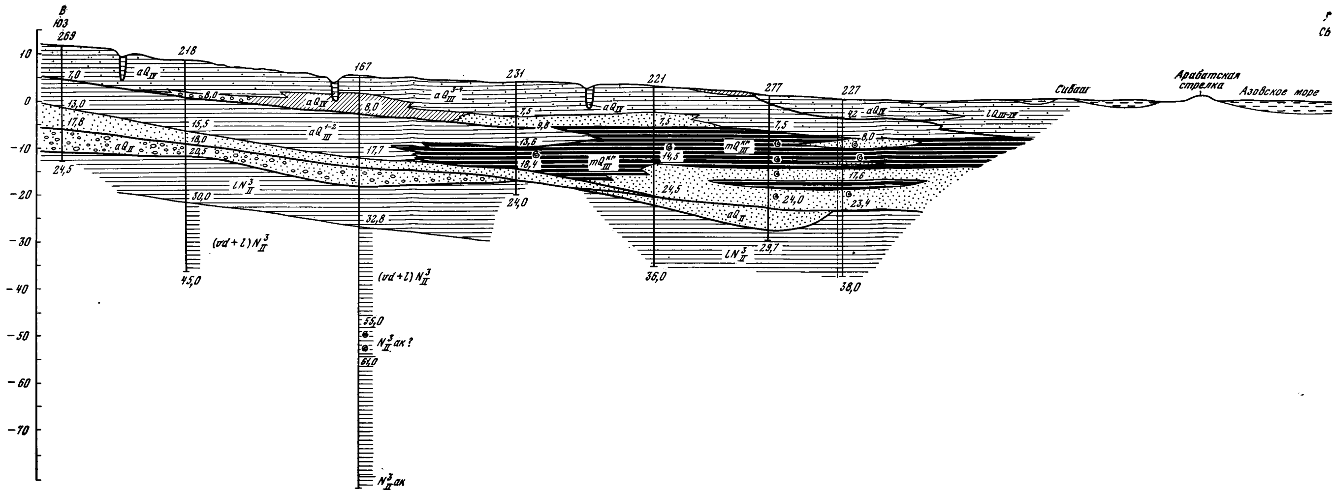
Рис. 3. Геологический разрез по линии В—Г Условные обозначения см. рис. 2.
