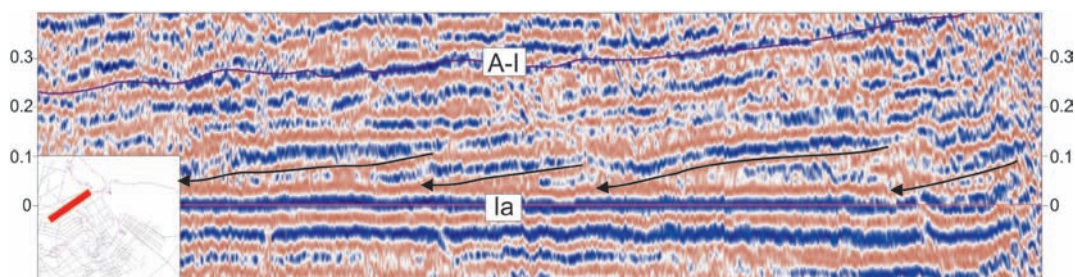
Рис. 6. Подошвенное прилегание пермских отложений к кровле карбонатов в акваториальной части Коротаихинской впадины
