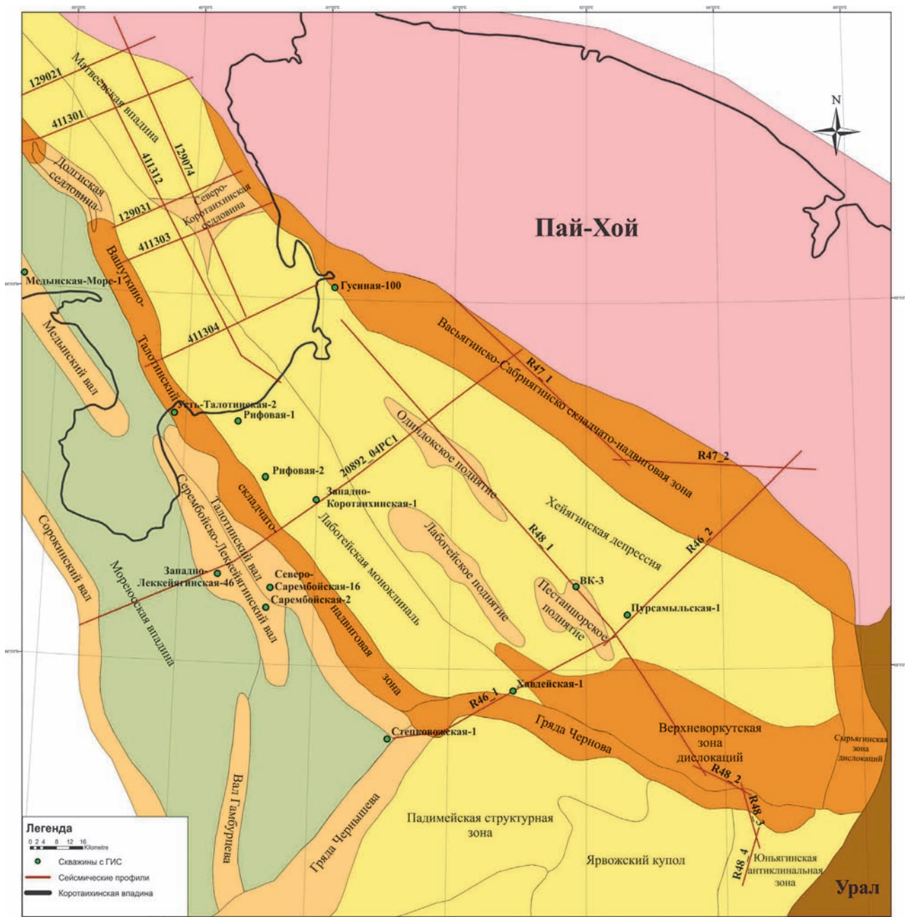
Рис. 1. Структурно-тектоническая схема Коротайхинской впадины
