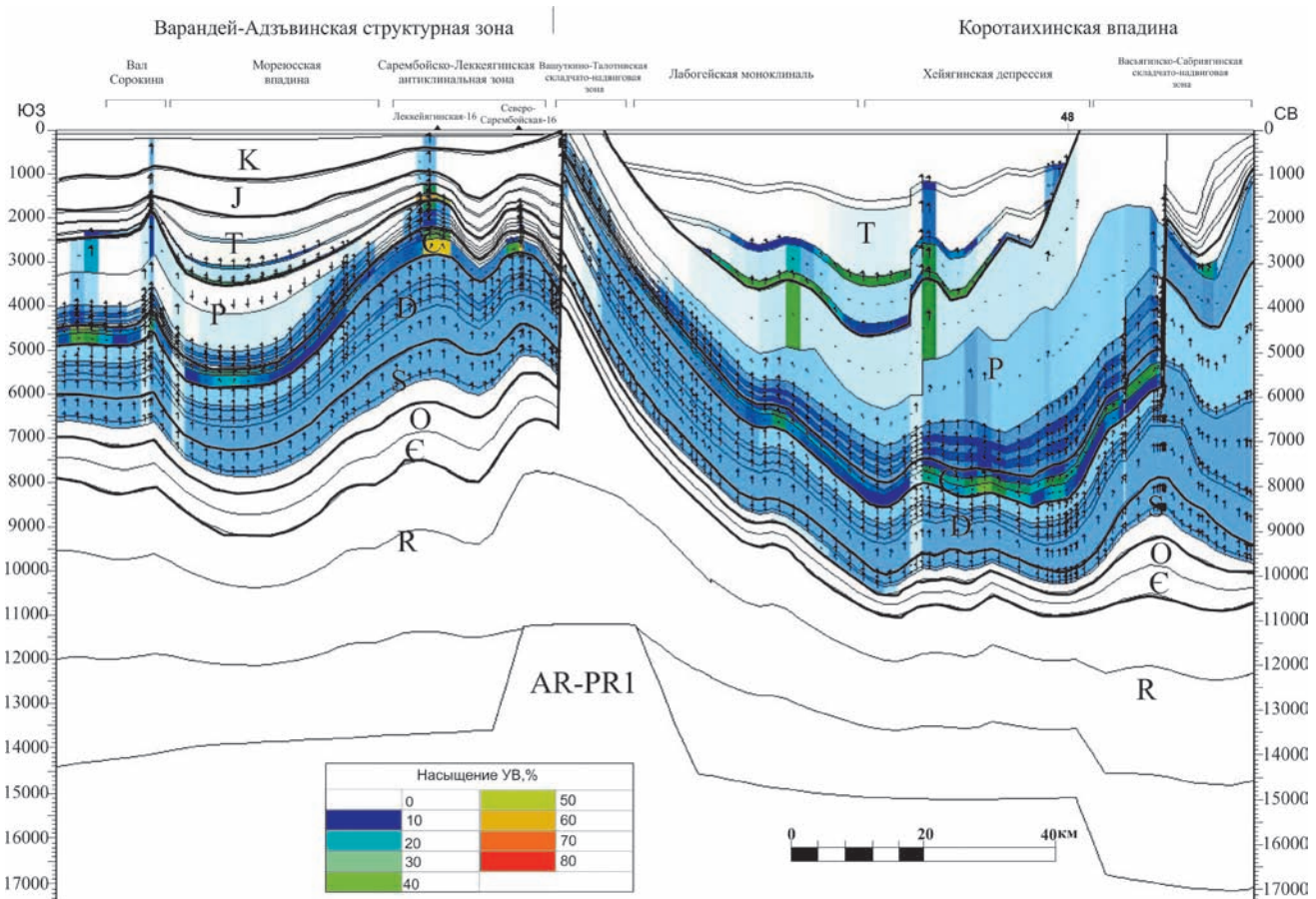
Рис. 13. Направление миграции и степень насыщения УВ. Профиль 20892-04P
