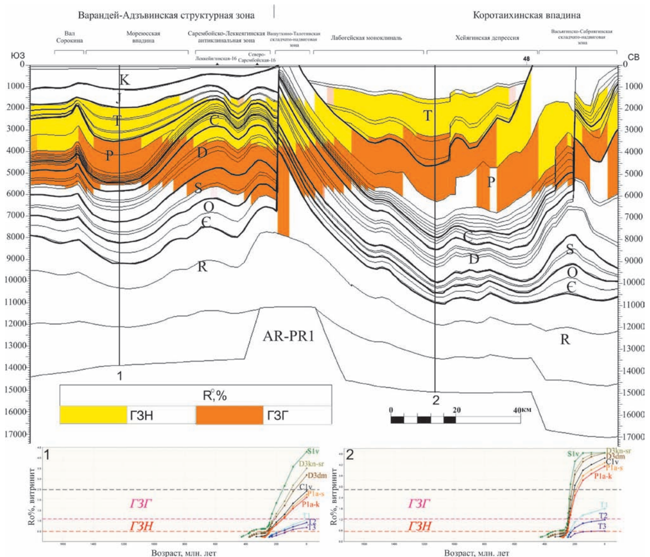
Рис. 12. Степень катагенетической преобразованности осадочной толщи. Профиль 20892-04РС1
