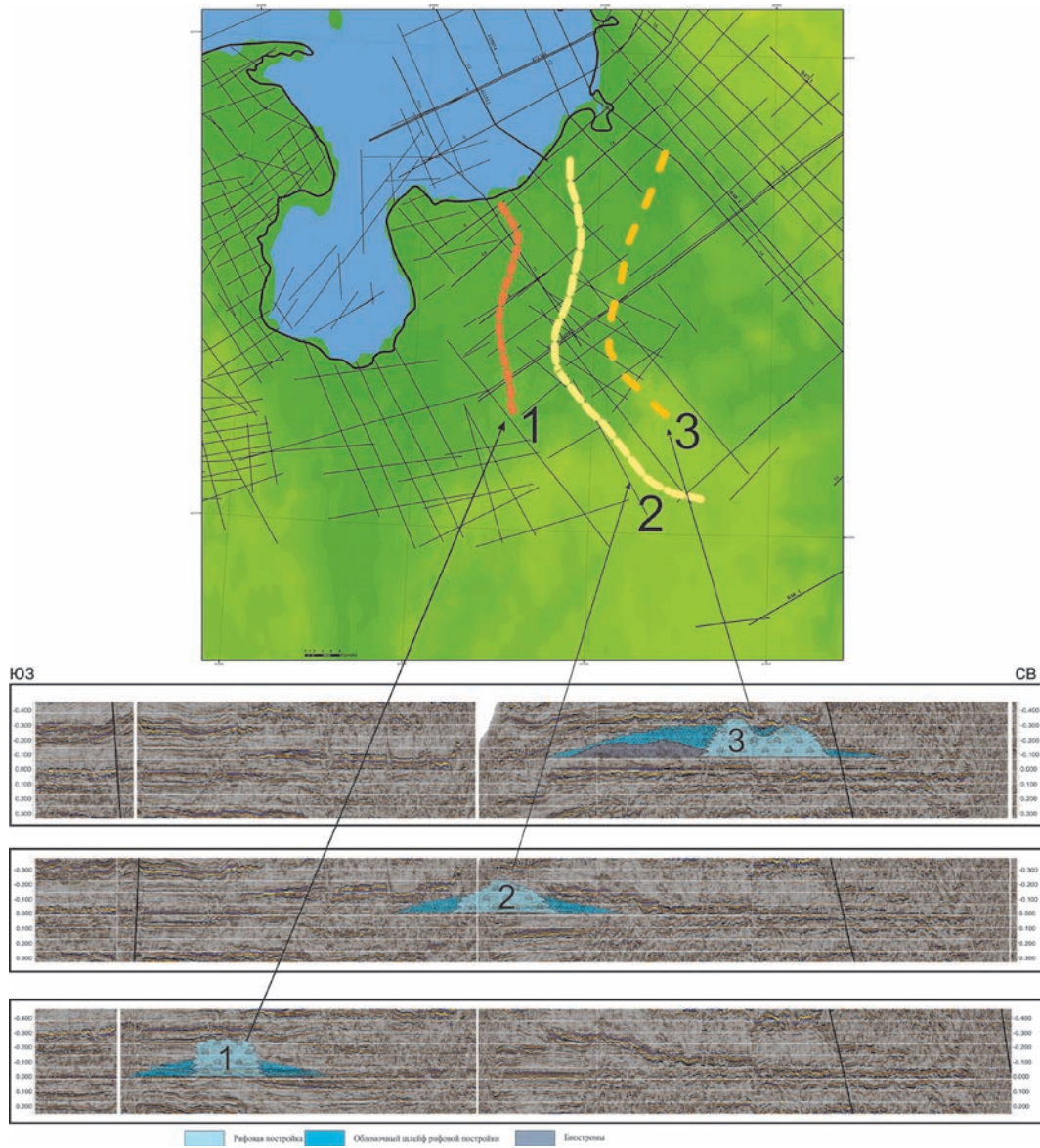
Рис. 4. Проградация рифовых тел на западном борту Коротаихинской впадины
