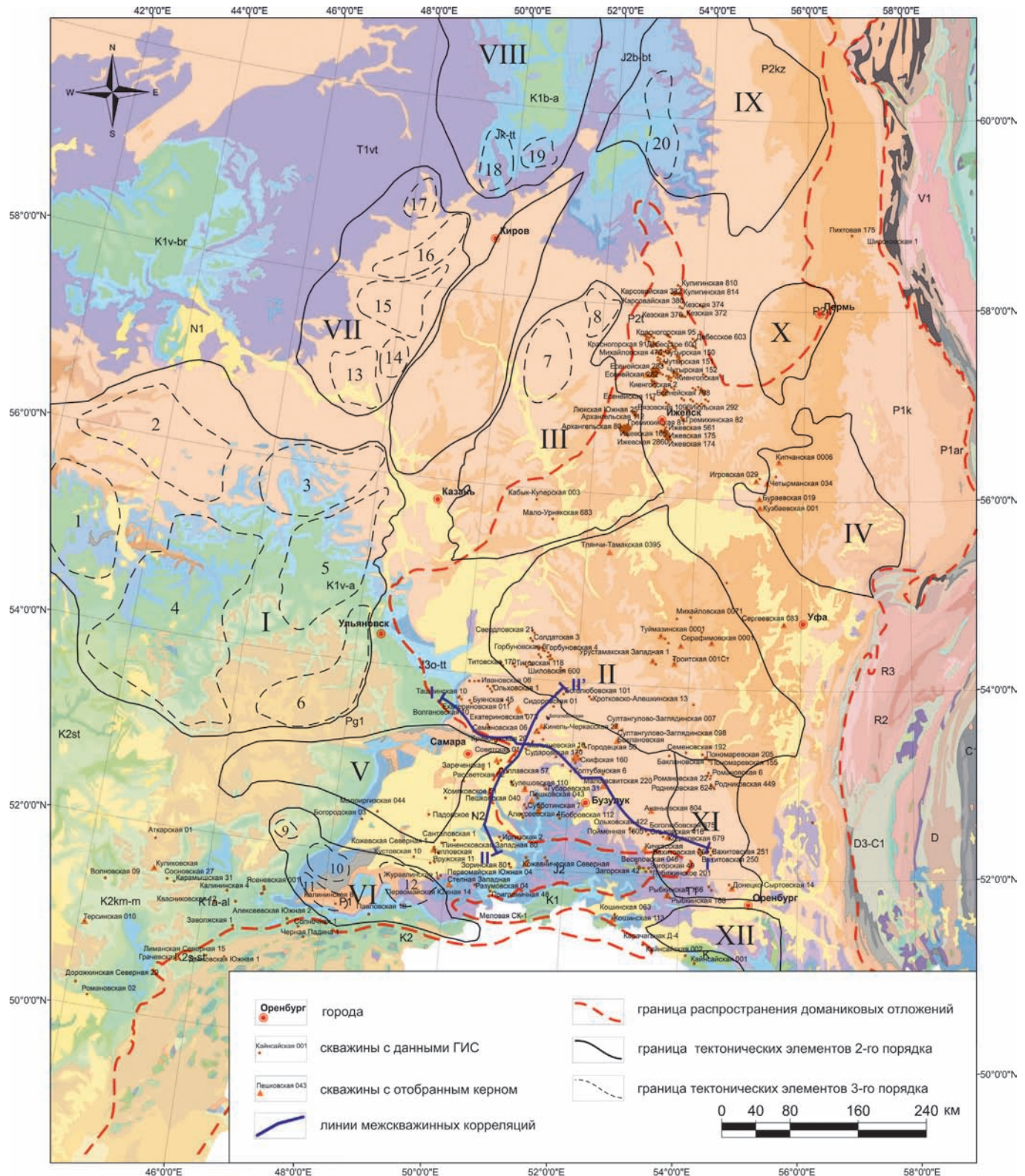
Границы крупных тектонических элементов: I - Токмовский свод, II - Южно-Татарский свод, III - Северо-Татарский свод, IV - Башкирский свод, V - Жигулевский свод, VI - Пугачевский свод, VII - Котельничский погребенный свод, VIII - Сыктывкарский огребенный свод, IX - Камский свод, X - Пермский свод, XI - Восточно-Оренбургское валообразное поднятие, XII - Соль-Илецкий Выступ. Границы средних тектонических элементов: 1 - Темниковская вершина, 2 - Нижегородская вершина, 3 - Сундырская вершина, 4 - Токмовская вершина, 5 - Канашская вершина, 6 - Ульяновская вершина, 7 - Ломикский купол, 8 - Ярский купол, 9 - Терешкинская вершина, 10 - Балаковская вершина, 11 - Марьевская вершина, 12 - Клиновская вершина, 13 - Санчурский выступ, 14 - Яранский выступ, 15 - Парфеновский выступ, 16 - Котельничский выступ, 17 - Даровский выступ, 18 - Летниковский выступ, 19 - Синегорский выступ, 20 - Лойнинский выступ.
