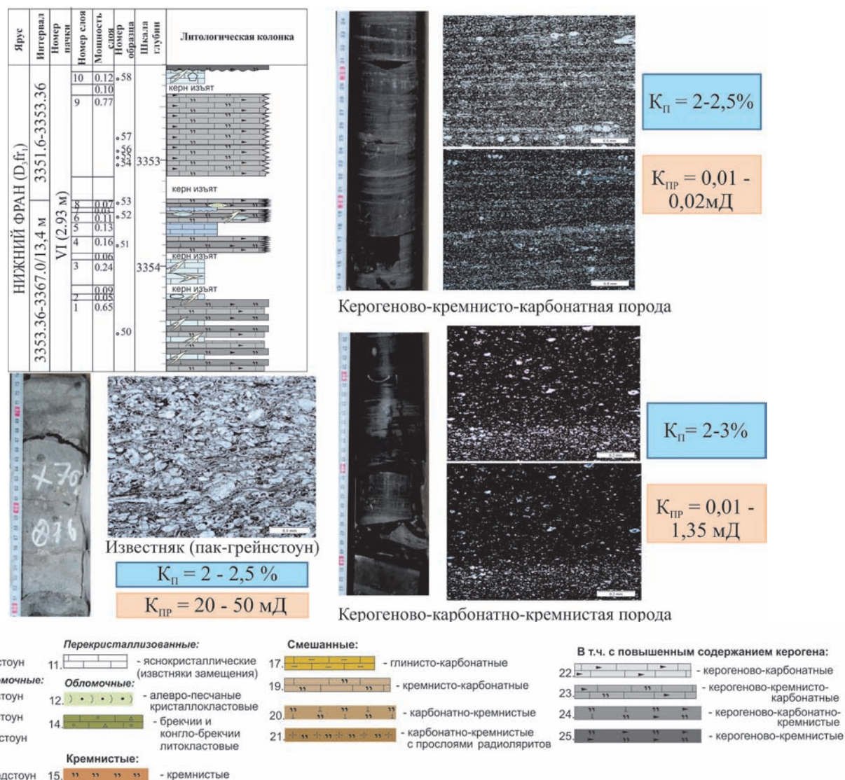
Рис. 7. Отложения относительно глубоководных внутришельфовых впадин
