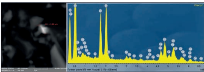
Рис. 4. Монацит (с РЗМ) в пробе угля Ланковского месторождения
