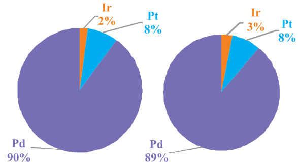
Рис. 5. Структура МПГ в углях (Корфское, Эльгенское и др. месторождения), а – Соотношение содержания металлов платиновой группы в углях Эльгенского месторождения, б – Соотношение содержания металлов платиновой группы в углях Корфского месторождения
