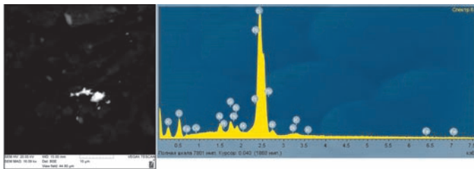
Рис. 3. Платиносодержащее включение в пробе угля Эльгенского месторождения
