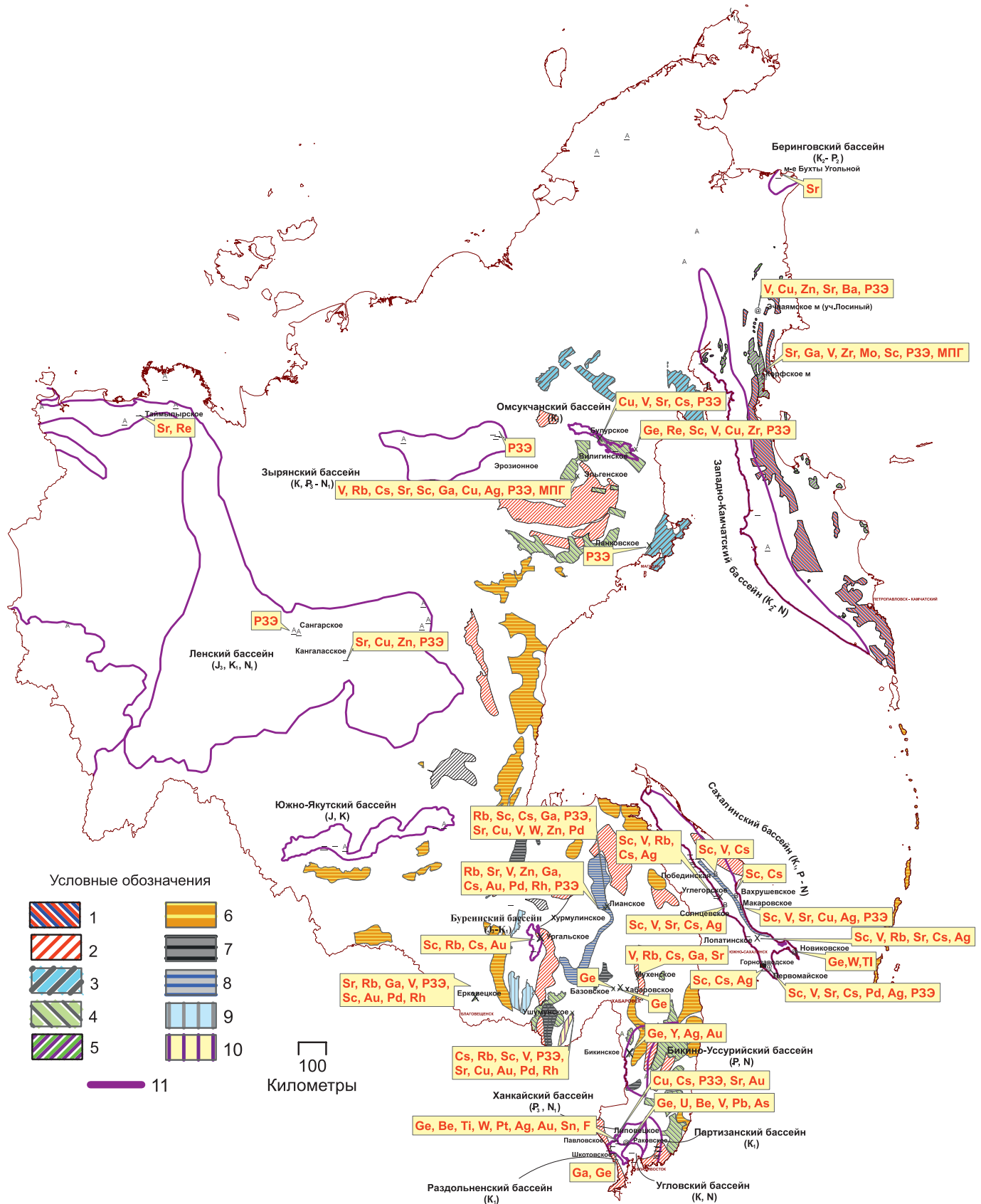
Рис. 9. Карта металлоносности угольных месторождений и бассейнов Дальневосточного ФО России на минерагенической основе. Профильный тип оруденения минерагенических таксонов: 1 – золото-серебряное эпitherмальное оруденение с полиметаллической минерализацией; 2 – существенно золотое оруденение: золото-кварцевое, золото-сульфидное, золото-сурьмяное, золото-вольфрамовое; 3 – медно-порфировое оруденение с золото-серебряной минерализацией; 4 – оловянное, вольфрамовое, олово-серебро-полиметаллическое оруденение жильного, скарнового, грейзенового типов; 5 – связанное с базит-ультрабазитовыми комплексами: хромитовое, платиновое, медно-никелевое оруденение; 6 – золото-серебряное эпitherмальное оруденение; 7 – марганцевое, железо-марганцевое, фосфор-железо-марганцевое осадочное оруденение; 8 – ртутное и сурьмяно-ртутное оруденение; 9 – существенно молибденовое (в том числе с Cu и Au) жильного, грейзенового, порфирового типов; 10 – редкометалльное, апатит-редкометалльное и редкоземельное оруденение карбонатитового и грейзенового типов. Границы: 11 – угольных бассейнов
