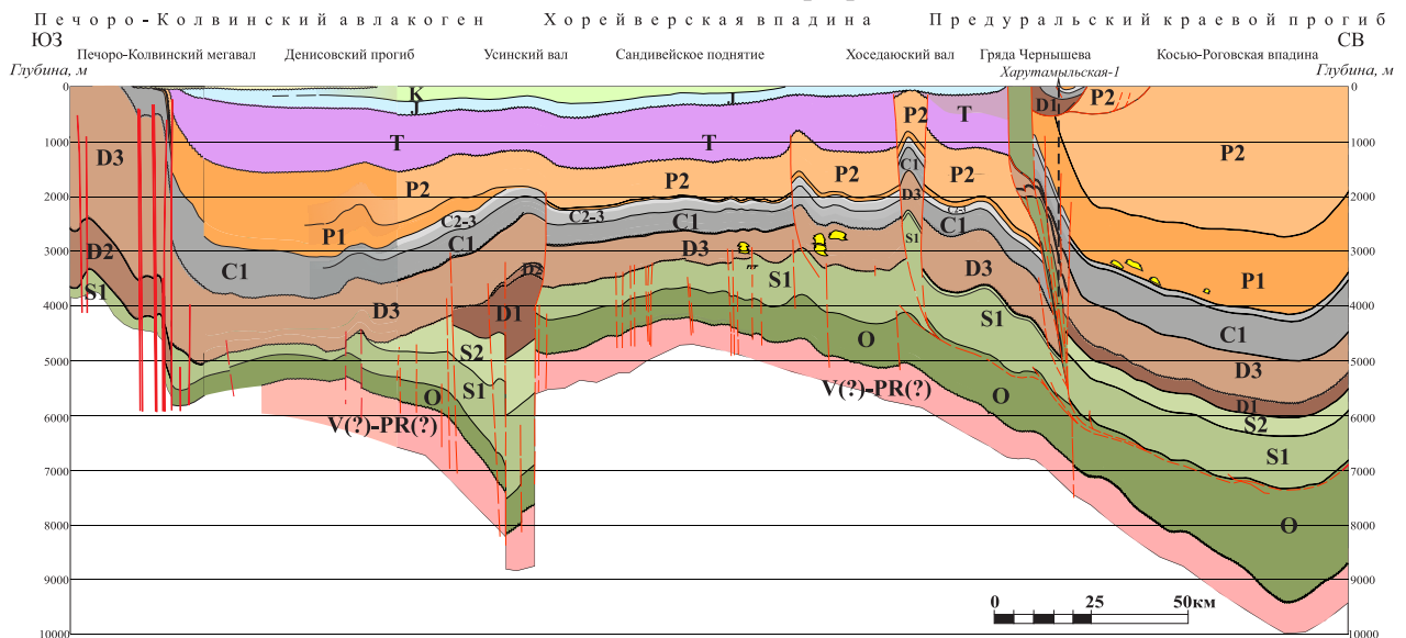
Рис. 5. Геологический разрез по линии профиля P-17 («Изучение и анализ ресурсной базы углеводородного сырья на территории Тимано-Печорской нефтегазоносной провинции»)
