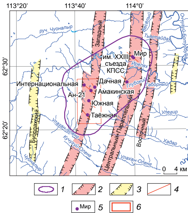
Рис. 2. ТЕКТОНИЧЕСКАЯ СХЕМА МИРНИНСКОГО КИМБЕРЛИТОВОГО ПОЛЯ:
