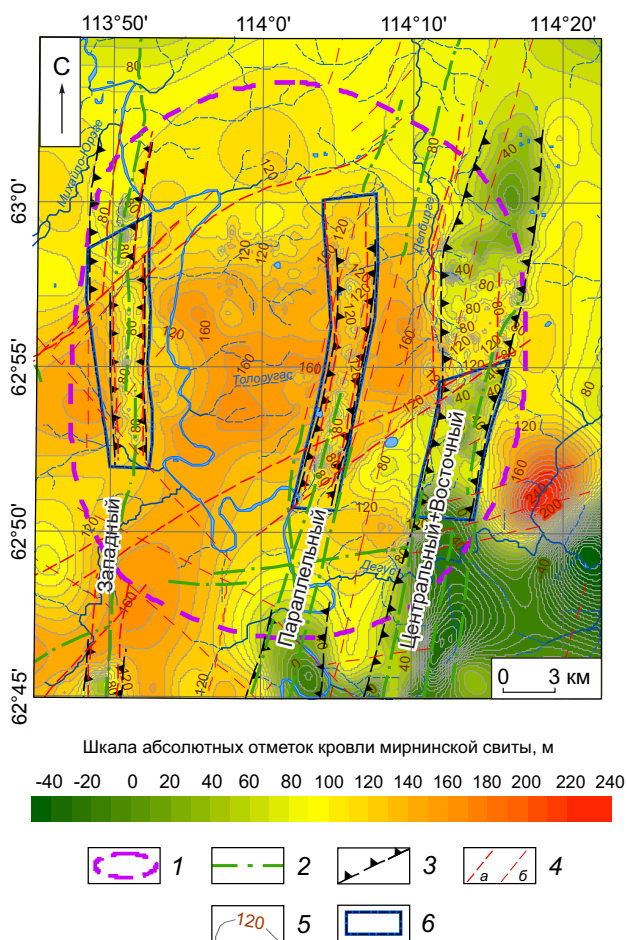
Рис. 7. СТРУКТУРНО-ТЕКТОНИЧЕСКАЯ КАРТА БАХЧИНСКОГО ПРОГНОЗИРУЕМОГО ПОЛЯ:
