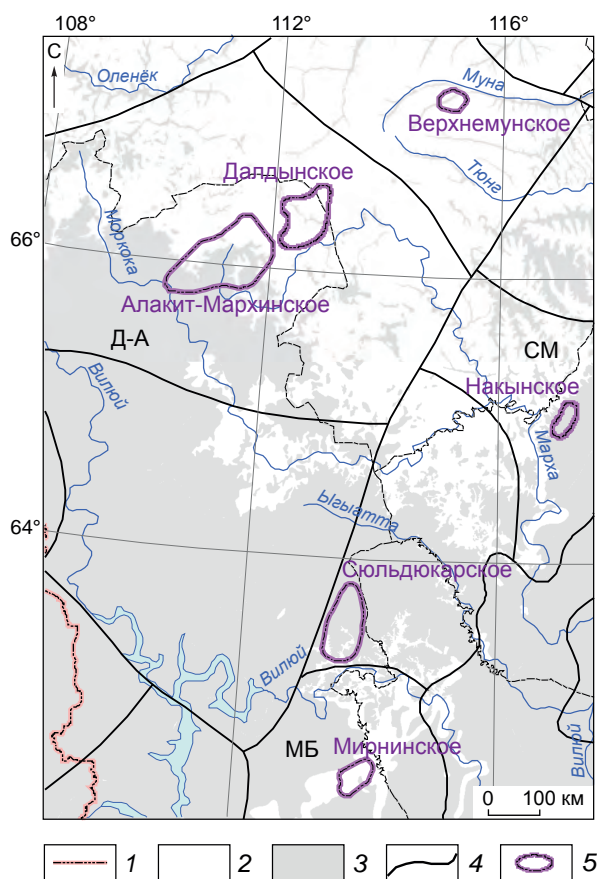
Рис. 1. МИНЕРАГЕНИЧЕСКАЯ СХЕМА ЦЕНТРАЛЬНО-СИБИРСКОЙ АЛМАЗОНОСНОЙ СУБПРОВИНЦИИ ЗАПАДНОЙ ЯКУТИИ:
