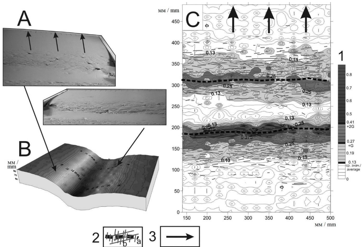
Рис. 1. Результаты физического моделирования зоны растяжения в упруго-пластичной модели: А – фотографии, отражающие особенности рельефа сбросовых зон над разными штампами установки «Разлом»; В – цифровая модель рельефа; С – распределение величин градиента вертикальных движений на поверхности модели в изолиниях 1 – шкала величин градиента вертикальных движений; 2 – разрывы, выделенные на поверхности модели (а – магистральный сместитель, b – сопутствующие разрывы); 3 – направление перемещения активного штампа установки «Разлом»
