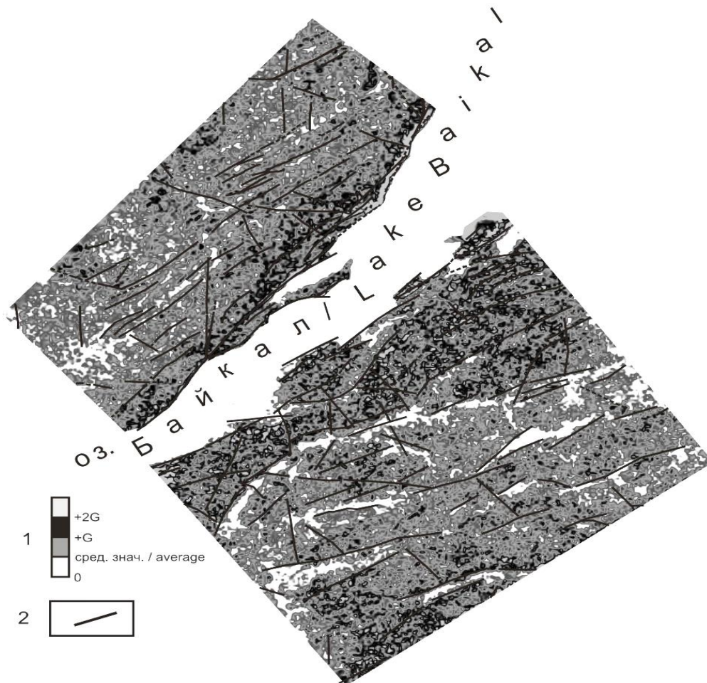
Рис. 3. Распределение градиента рельефа для СЗ и ЮВ флангов Байкальского рифта с разноранговыми линеаментами: 1 – шкала величин градиента рельефа (уровень среднего значения, стандартного и двух стандартных отклонений); 2 – крупные линеаменты Fig. 3. Relief gradient distribution for the north-west and south-east flanks of the Baikal rift with different rank lineaments: 1 – scale of relief gradient values (level of the mean, standard and two standard deviations); 2 – large lineaments
