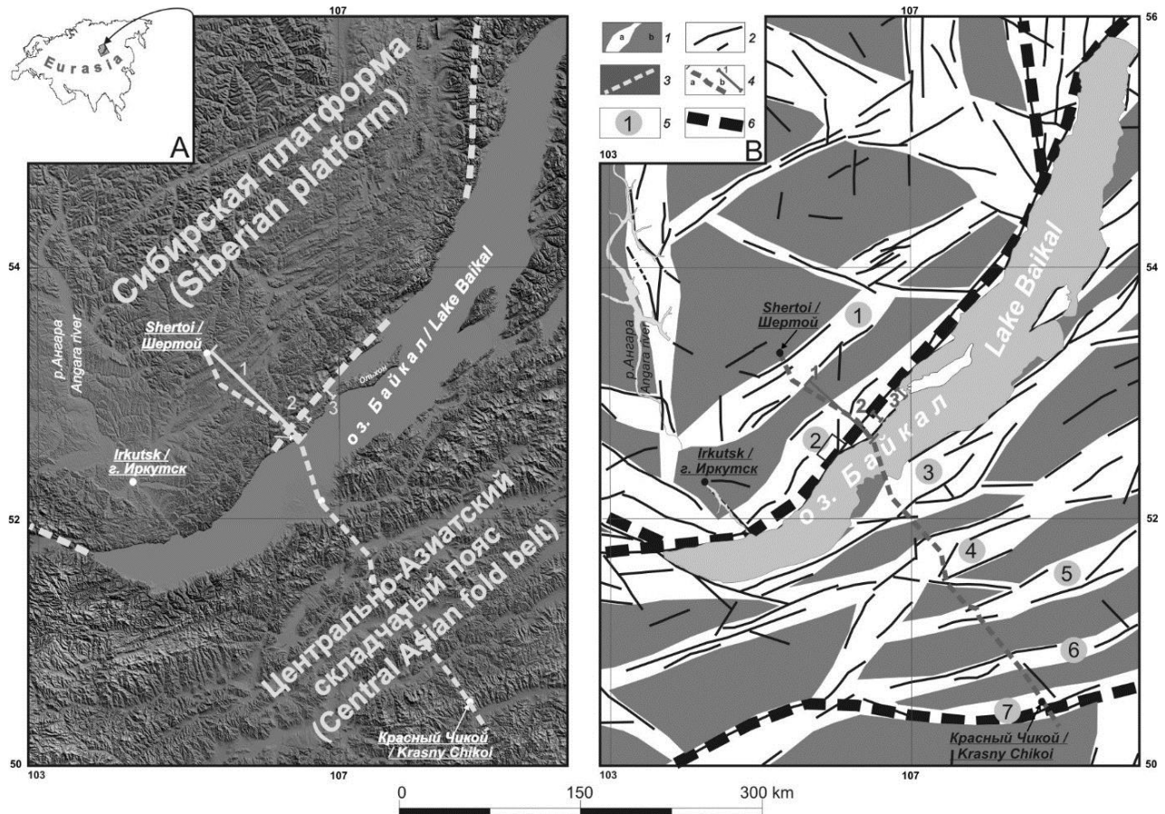
Рис. 2. Трехмерная модель рельефа (А) и построенная на ее основе схема зонно-блоковой структуры земной коры (В) Прибайкалья и Западного Забайкалья [2]:
