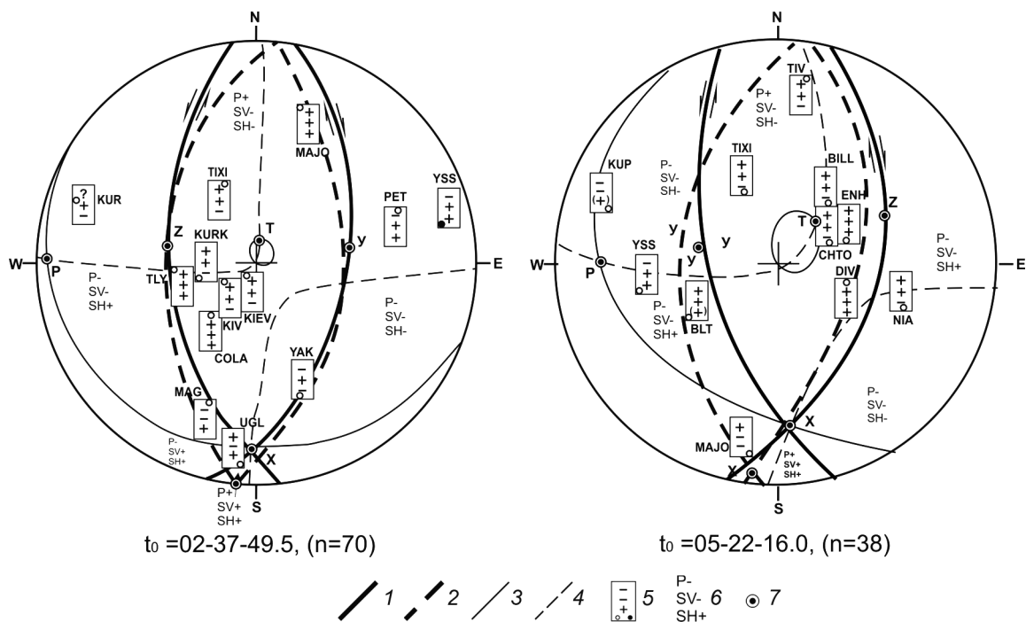
Рис. 3. Стереогаммы механизмов очагов Невельских землетрясений 2 августа 2007 г. с MLH \geq 6.0 . (верхняя полусфера). 1–2 – положение нодальных плоскостей решений ИМГ и Г ДВО РАН (настоящая работа) и GCMТ, соответственно; 3–4 – нодальные линии SV = 0 и SH = 0 , соответственно; 5–6 – экспериментальные (5) и теоретические (6) знаки первых смещений в волнах P , SV , SH (пустой кружок соответствует волне, распространявшейся от очага вниз, зачерненный – волне, распространявшейся от очага вверх); 7 – положение осей P , T , X , Y , Z для решений механизма, согласованных со знаками в P , PG , S , SG -волнах.
