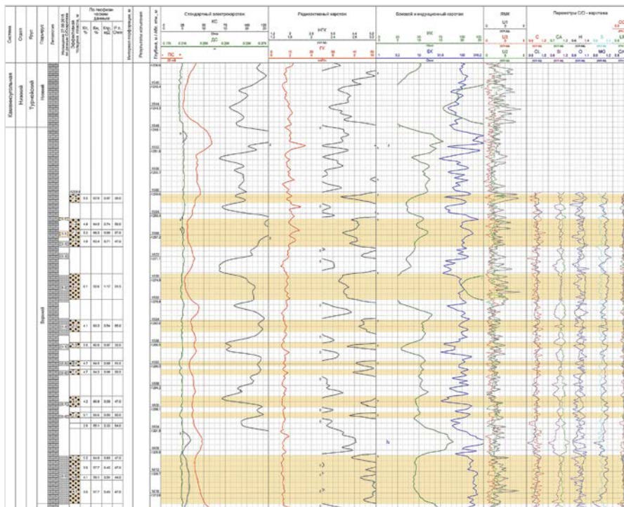
Рис. 4 — Фрагмент геолого-геофизического разреза доманиковых отложений по скважине №411 (Бухараевское месторождение)
