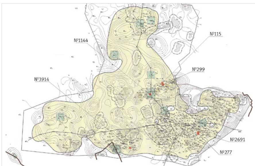
Рис. 3 — Скважины, в которых был проведен ИННК (С/О-каротаж) (Бавлинское месторождение)
