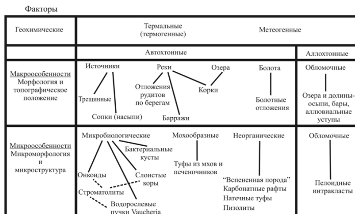
Рис. 2. Объединенная схема классификации травертинов по [27].
