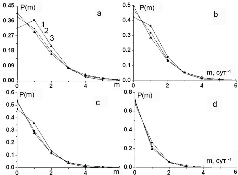
Рис. 6. То же, что на рис.5, но для каталога KNET.
