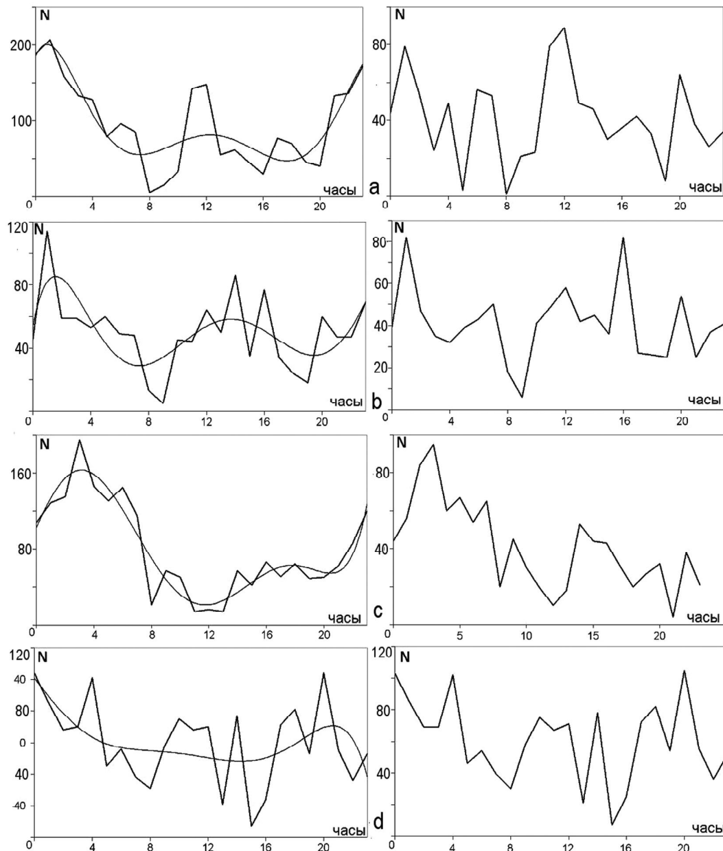
Рис. 2. Суточные распределения количества сейсмических событий ( N ) для исследуемых субрегионов.
