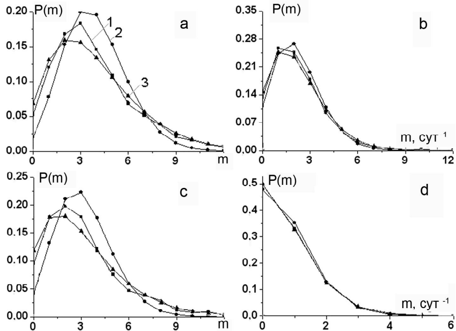
Рис. 5. Графики распределения событий по числу m событий за сутки (1), с нормировкой на полное число событий для выборок из каталога KAZ.
