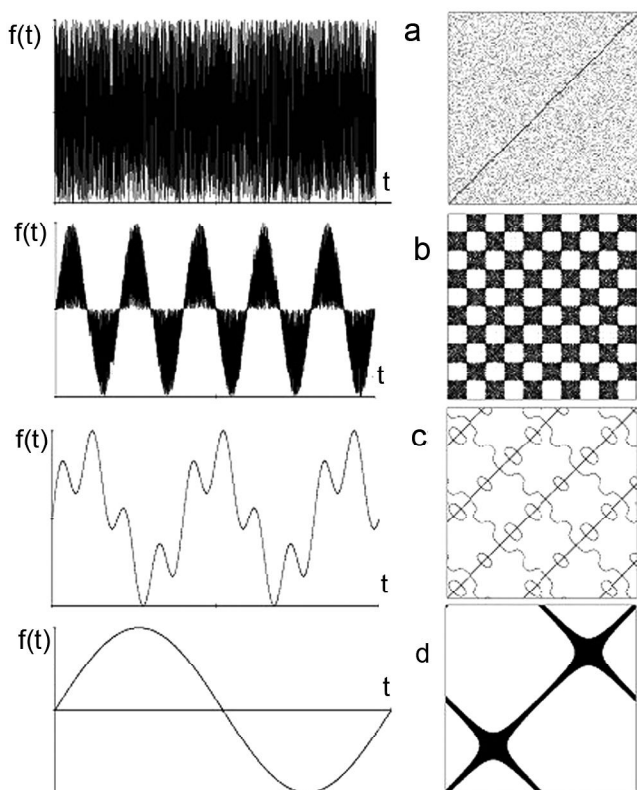
Рис. 3. Тестовые сигналы и вид рекуррентных диаграмм.
