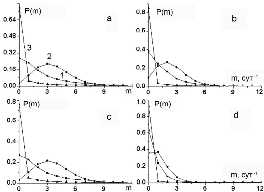
Рис. 7. То же, что на рис. 5, но для каталога южной части о. Сахалин.
