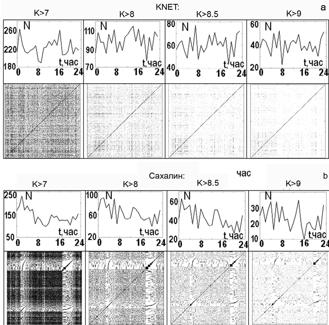
Рис. 4. Распределения числа событий по времени суток и рекуррентные диаграммы для выборок по превышению энергетического порога (нижней граница).
