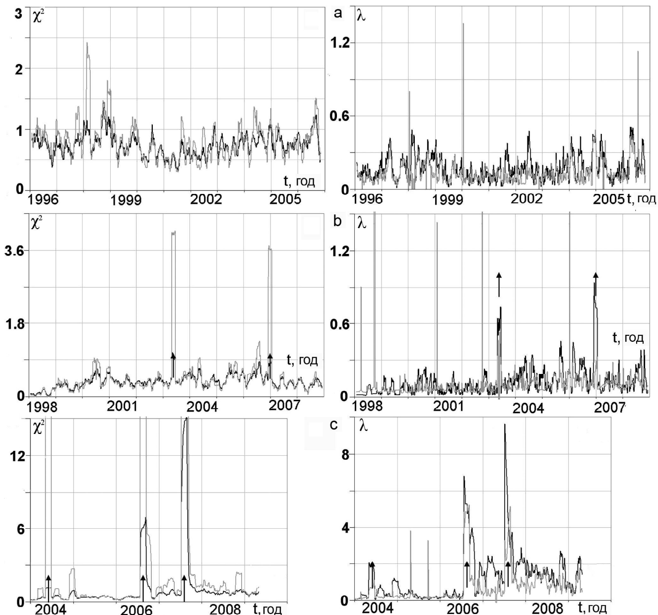
Рис. 8. Изменения параметра соответствия эмпирического распределения сейсмичности рассматриваемых регионов с распределениями Пуассона (черная линия) и Пойа (серая линия) по критериям Пирсона ( \chi^2 ), и Колмогорова-Смирнова ( \lambda ) для каталогов.
