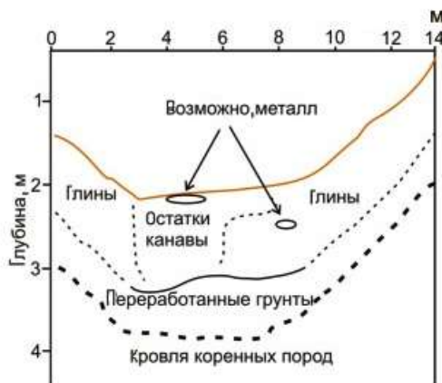
Рисунок 4. Результаты обработки и интерпретации по профилю 8. Figure 4. Results of processing and interpretation according to profile 8.
