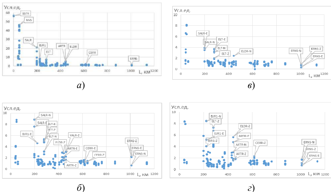
Рис. 3. Графики отношений амплитуд монохромов к среднеквадратическим амплитудам шумов в диапазоне 6-12 Гц в зависимости от удалений:
