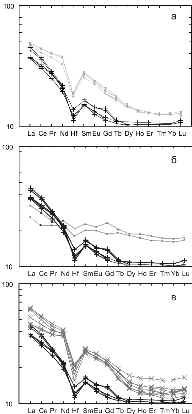
Рис. 13. Сопоставление нормализованных к хондриту спектров распределения редкоземельных элементов и Hf в «адакитоподобной» тефре о. Матуа и базальтах влк. Алайд северного звена Курильской гряды (а), тыловодужных лавах южных островов (б) и в океанических осадках скважин глубоководного бурения 579 и 581 (в).
