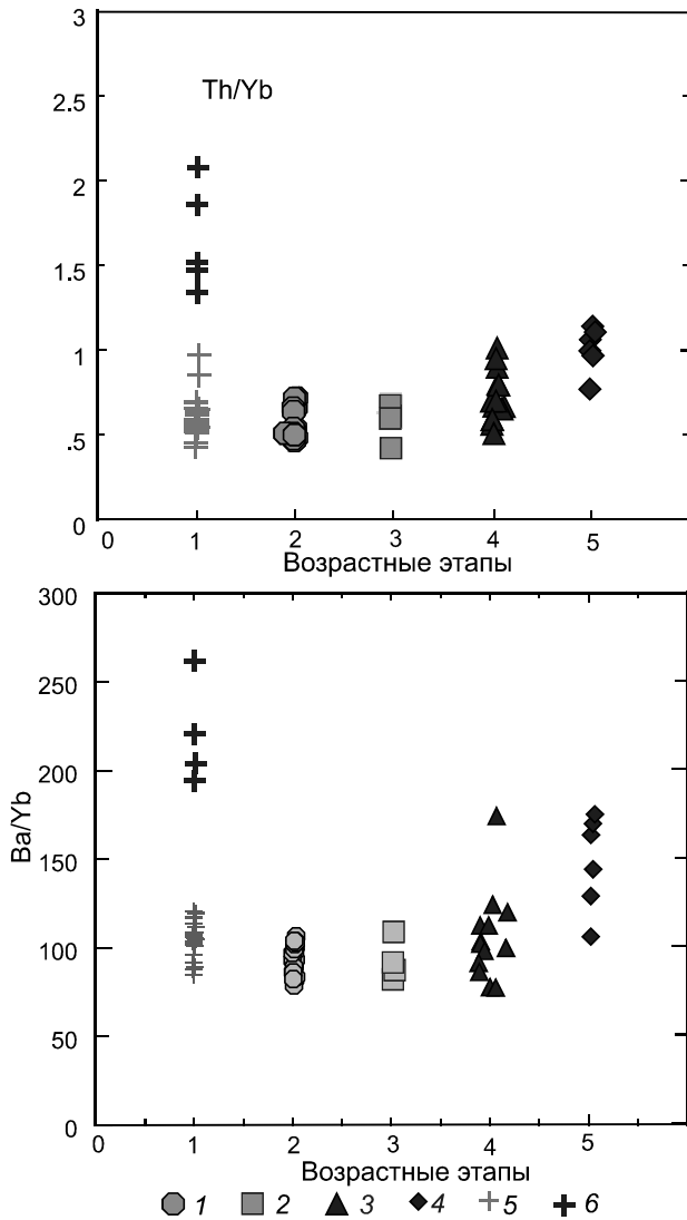
Рис. 11. Вариации отношений Ba/Yb и Th/Yb, Zr/Hf в основных вулканитах о. Матуа.
