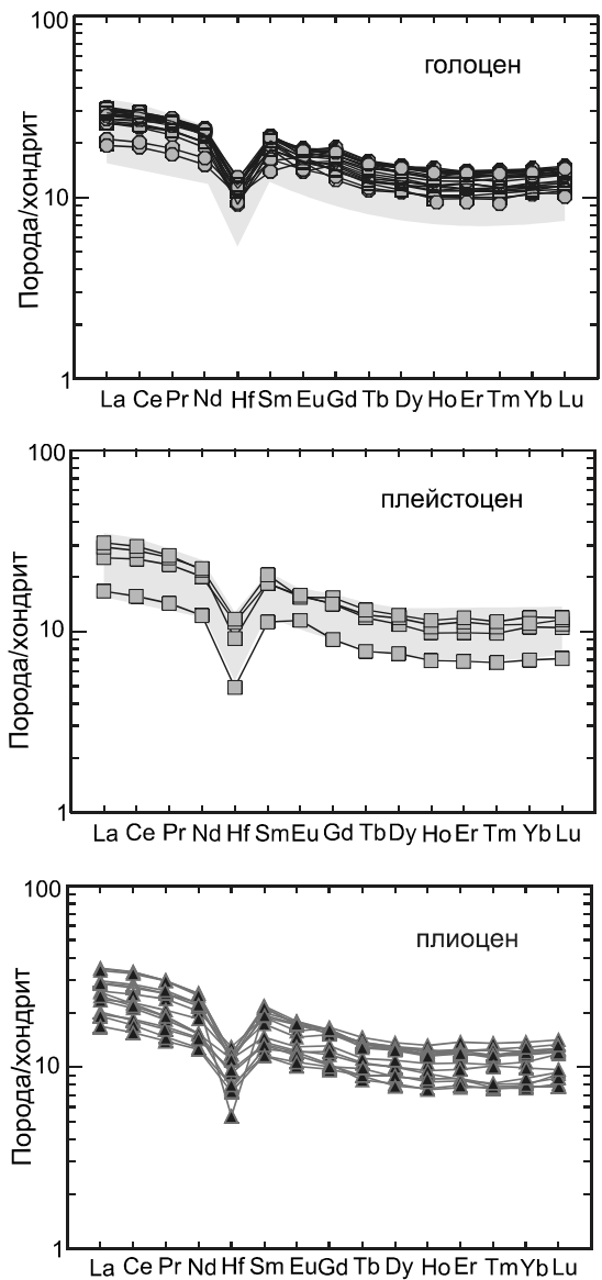
Рис. 7. Нормализованное к хондриту распределение редкоземельных элементов и Hf в разновозрастных вулканиках о. Матуа.
