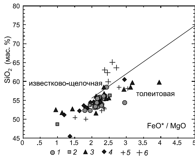
Рис. 3. Классификационная диаграмма \text{SiO}_2\text{--FeO}^*/\text{MgO} . Условные обозначения см. рис. 2.
