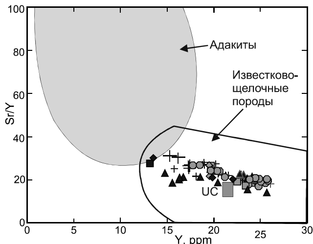
Рис. 10. Диаграмма Sr/Y–Y [19] для вулканогенных образований о. Матуа.
