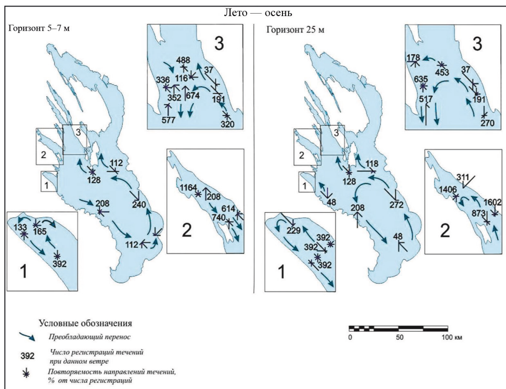
Рис. 8. Течения по данным длительных измерений при ветрах северных румбов (преобладающий ветер юго-восточного направления) (Филатов и др., 2010)
