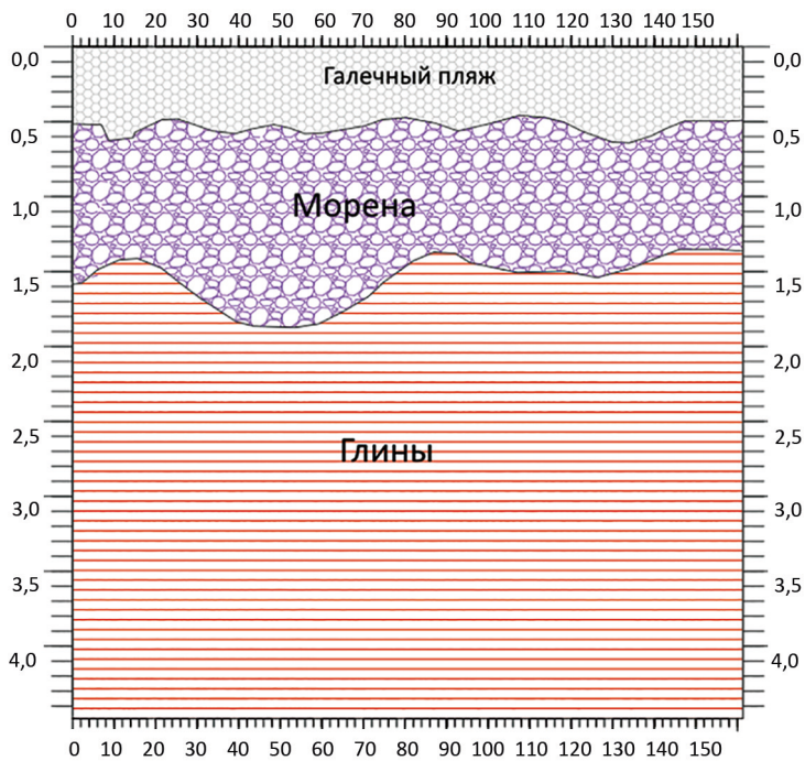
Рис. 4. Георадиолокационный профиль берега в районе Андомской горы
