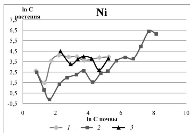
Рис. 5. Графики зависимости логарифмов содержаний Ni (ln C, мг/кг) в живой массе мхов от его содержания в почве в различных природно-техногенных условиях: 1 – лесные мхи в области аэрального загрязнения вблизи рудовозных дорог; 2 – болотные мхи в зоне окисления руд; 3 – мхи пойм рек ниже их пересечения рудовозными дорогами.
