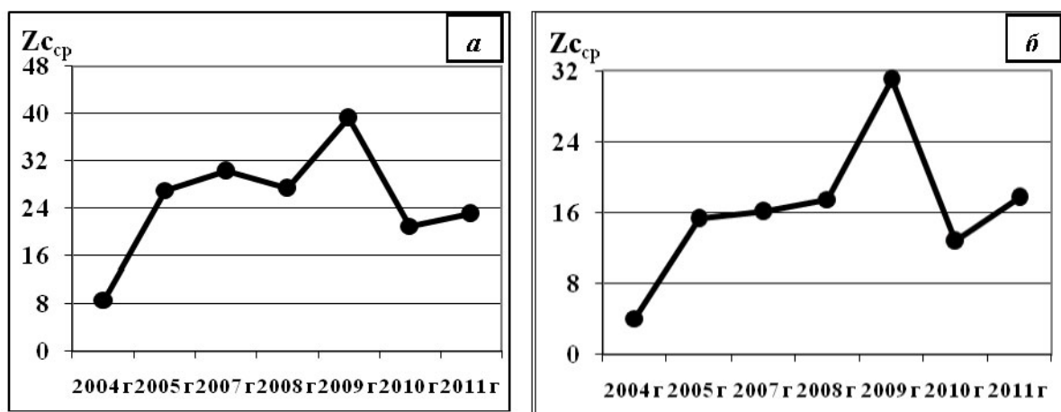
Рис. 3. Динамика изменений среднего значения суммарного показателя загрязнения Z_{c,cp} для почв (А) и мхов (Б) территории Шанучского рудника в период с 2004 по 2011 гг.
