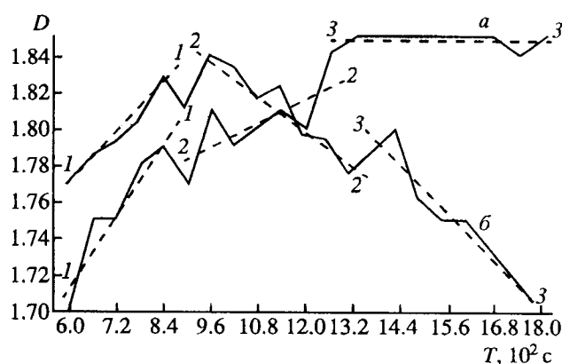
Рис. 2. Изменение фрактальной размерности D во времени T для всей совокупности разрывов в деструктивной зоне сдвига (а) и только для активных разрывов (б).
