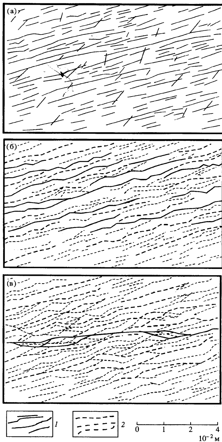
Рис. 1. Структурные схемы деструктивной зоны сдвига в первую (а), вторую (б) и третью (в) стадии её развития. 1 – активные разрывы; 2 – разрывы, утратившие активность.
