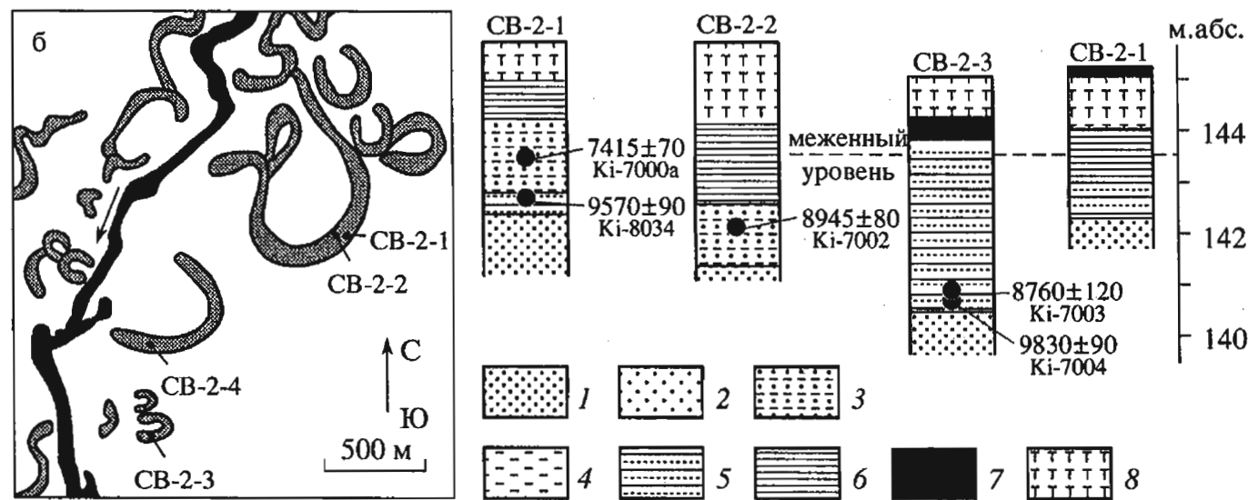
Рис. 6. Геологическое строение малых палеорусел (а – в долине Сейма (рис. 2), б – в долине Свапы (рис. 3)) 1 – песок среднезернистый; 2 – песок мелкозернистый; 3 – песок мелкозернистый заиленный (супесь); 4 – алевроит, легкий суглинок; 5 – глина опесчаненная, глина с песчаными прослоями; 6 – тяжелый суглинок, глина; 7 – сапропель; 8 – торф
