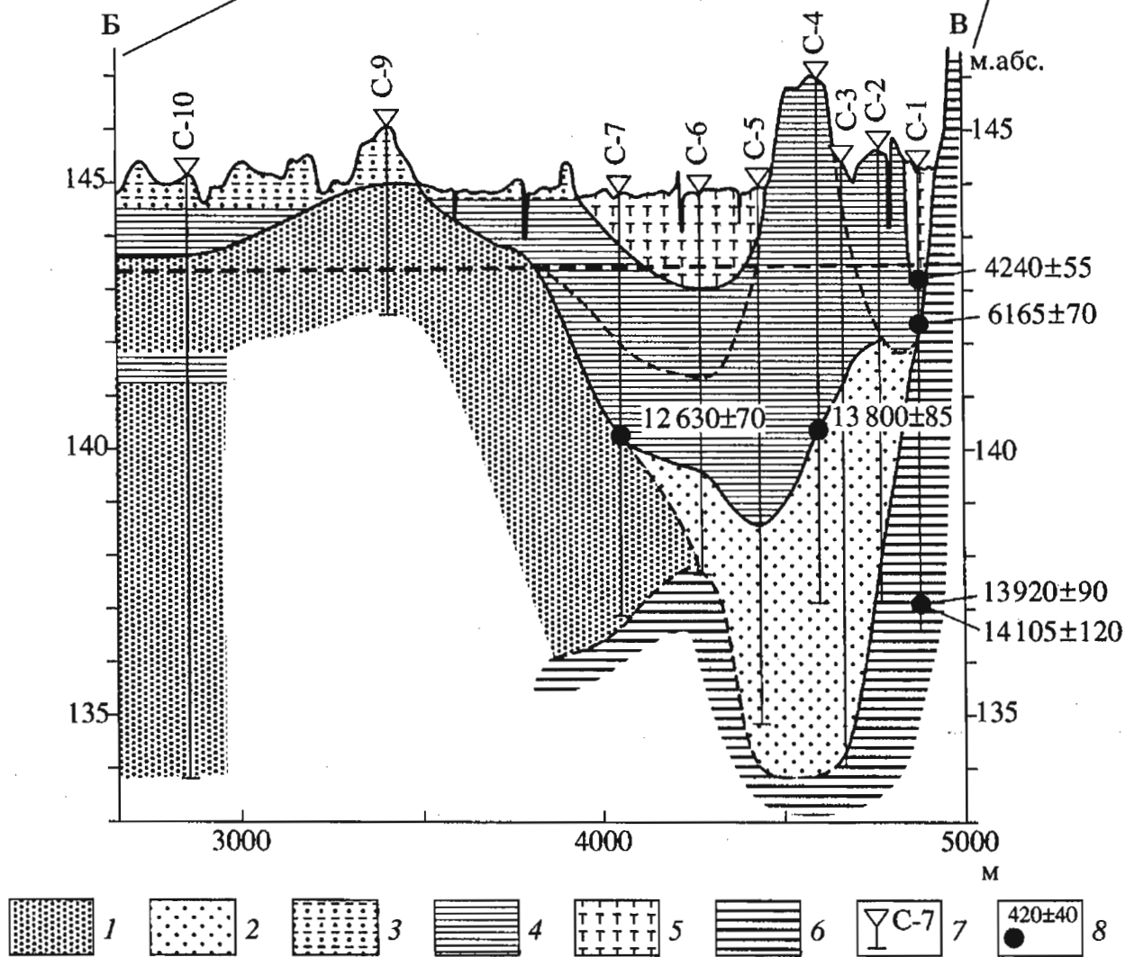
Рис. 4. Геологический профиль через палеорусл поздневалдайской макроизлучины Сейма у дер. Кудинцево (положение профиля – см. рис. 2)
