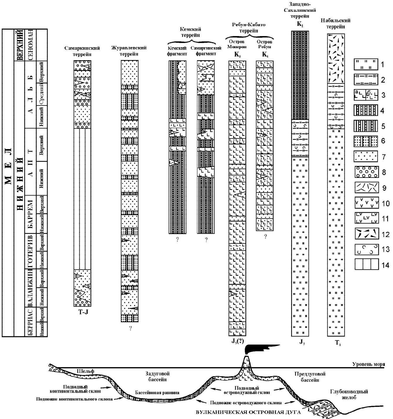
Рис. 5. Схема корреляции отложений различных латеральных элементов раннемеловой Монероно-Самаргинской островодужной системы.
