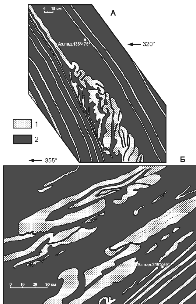
Рис. 4. Микрооползневые складки в верхней подсвите кемской свиты (левый берег руч. Холмогорка). Крылья синклинали: А – северо-западное (пачка 13, разрез VII), Б – юго-восточное (пачка 11, разрез VIII). Зарисовки обнажений.
