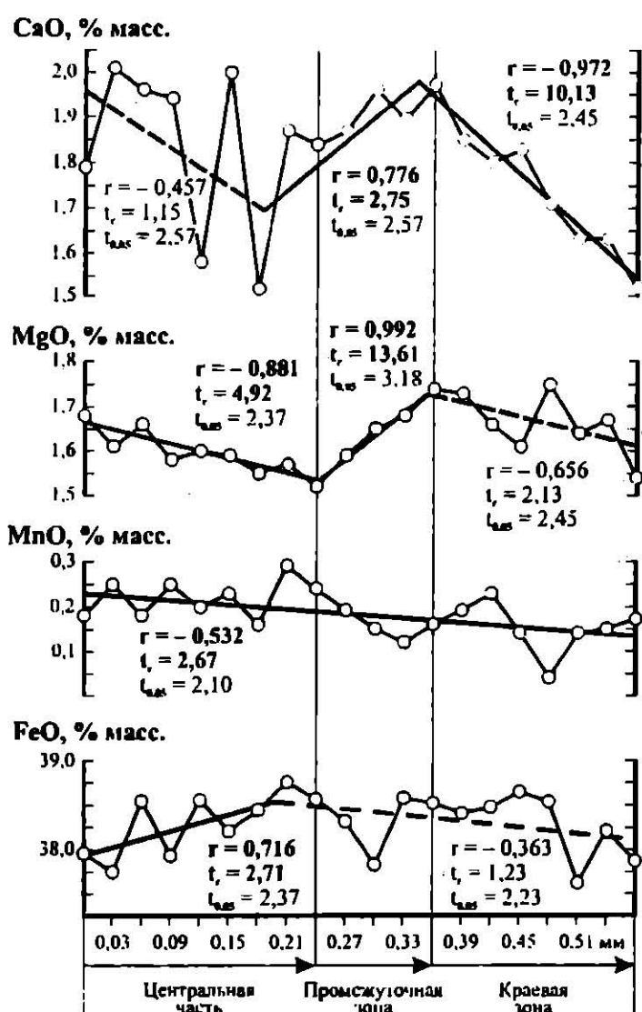
Рис. 3. Характер распределения компонентов в кристалле граната. Условные сокращения: Хср. – среднеарифметическое содержание компонента, r – коэффициент корреляции
