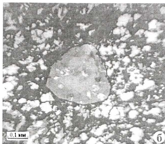
Рис. 2. Идиобластические кристаллы граната (а) и турмалина (б) в ороговикованном сланце ксенолита. Фото в проходящем поляризованном свете без анализатора. На зерне граната показан профиль микрозондовых анализов, приведенных в табл. 1
