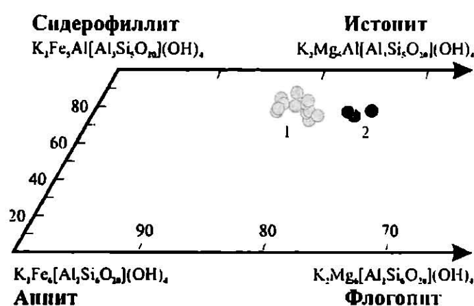
Рис. 4. Компонентный состав биотитов в ороговикованном гранат-биотитовом сланце ксенолита. Условные обозначения: 1 – на удалении от зерен турмалина, 2 – вблизи зерен турмалина
