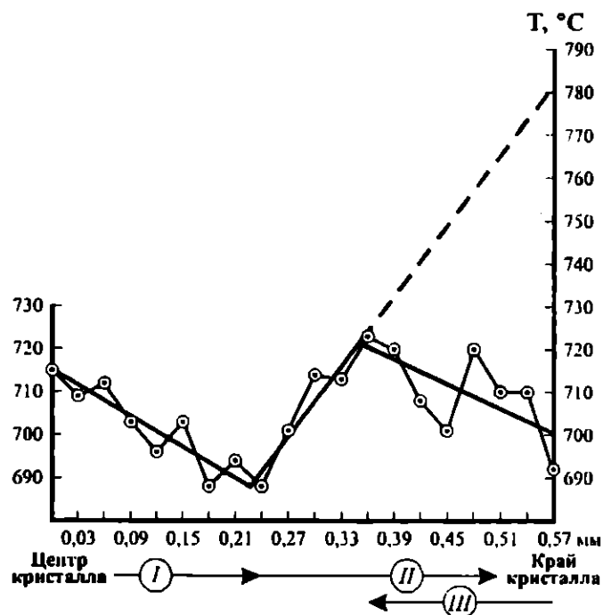
Рис. 5. Температурные условия кристаллизации различных зон роста идиобласт граната. Стадии: I – термальный метаморфизм в контактовом ореоле интрузии, II – метаморфические преобразования ксенолита в сиенитовом расплаве, III – регрессивные изменения при аутометаморфизме интрузивных пород
