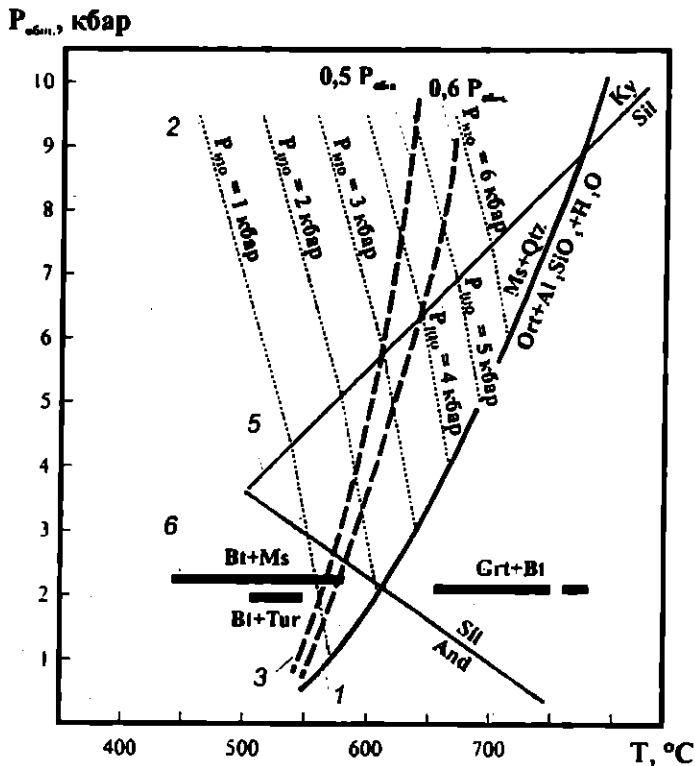
Рис. 6. Экспериментальные и расчетные кривые распада мусковита в присутствии кварца при различных соотношениях P_{общ.} и P_{H_2O} и равновесия в системе And - Ky - Sil [по 4 с изменениями]. Условные обозначения: 1-3 – моновариантные линии реакций разложения мусковита в присутствии кварца: 1 – по экспериментальным данным при P_{общ.} = P_{H_2O} [5,6]; 2 – при фиксированных значениях P_{H_2O} ; 3 – при P_{H_2O} = 0,5 и 0,6 P_{общ.} [7]; 4 – линия полиморфных переходов силикатов глинозема и координаты тройной точки по [8]; 5 – температурные оценки биминеральных равновесий в ксенолите Шебекинского массива
