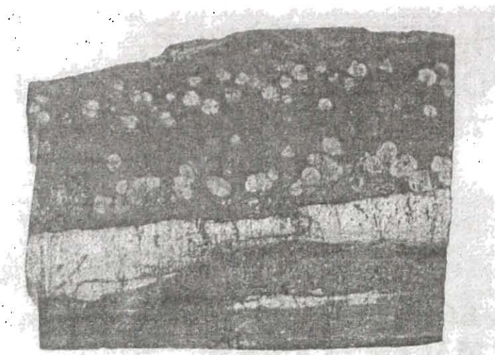
Рис. 1. Фрагмент ксенолита гранат-биотит-кварцевого ороговикованного сланца с прослоями кварцита. Нат. вел.
