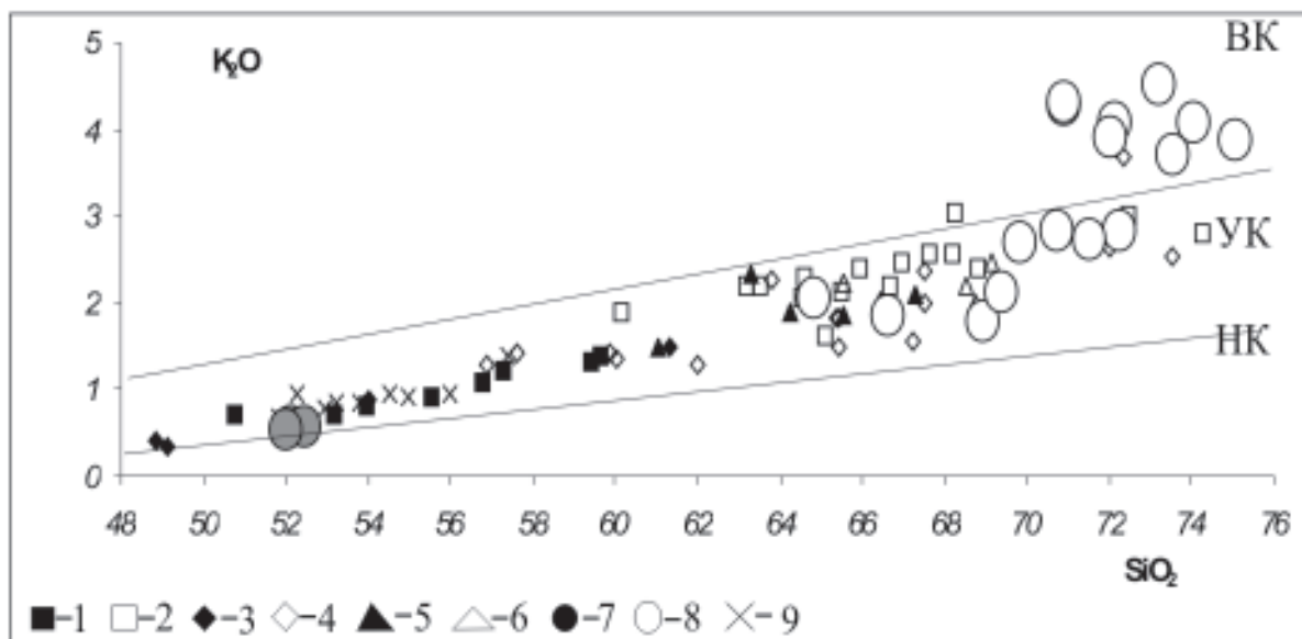
Рис.4. Диаграмма калиевости пемзовых бомб извержения 1996 г. в кальдере Академии Наук: НК – низкокальеиые, УК – умереннокальеиые, ВК – высококальеиые. Продукты извержений: 1 – влк. Однобокого, 2 - кальдеры Однобокого, 3 - влк. Половинка, 4 - к. Половинка, 5- влк. Академии Наук, 6 - к. Академии Наук, 7 – базальтовая тефра к. Академии Наук 1996 г., 8 - пемзовые бомбы к. Академии Наук 1996 г., 9 - базальтовая тефра прошлых извержений.
