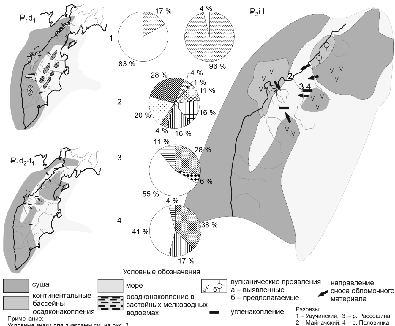
Рис. 10. Палеогеографическая схема центральной части Западной Камчатки для ипрско-лютетского времени.
