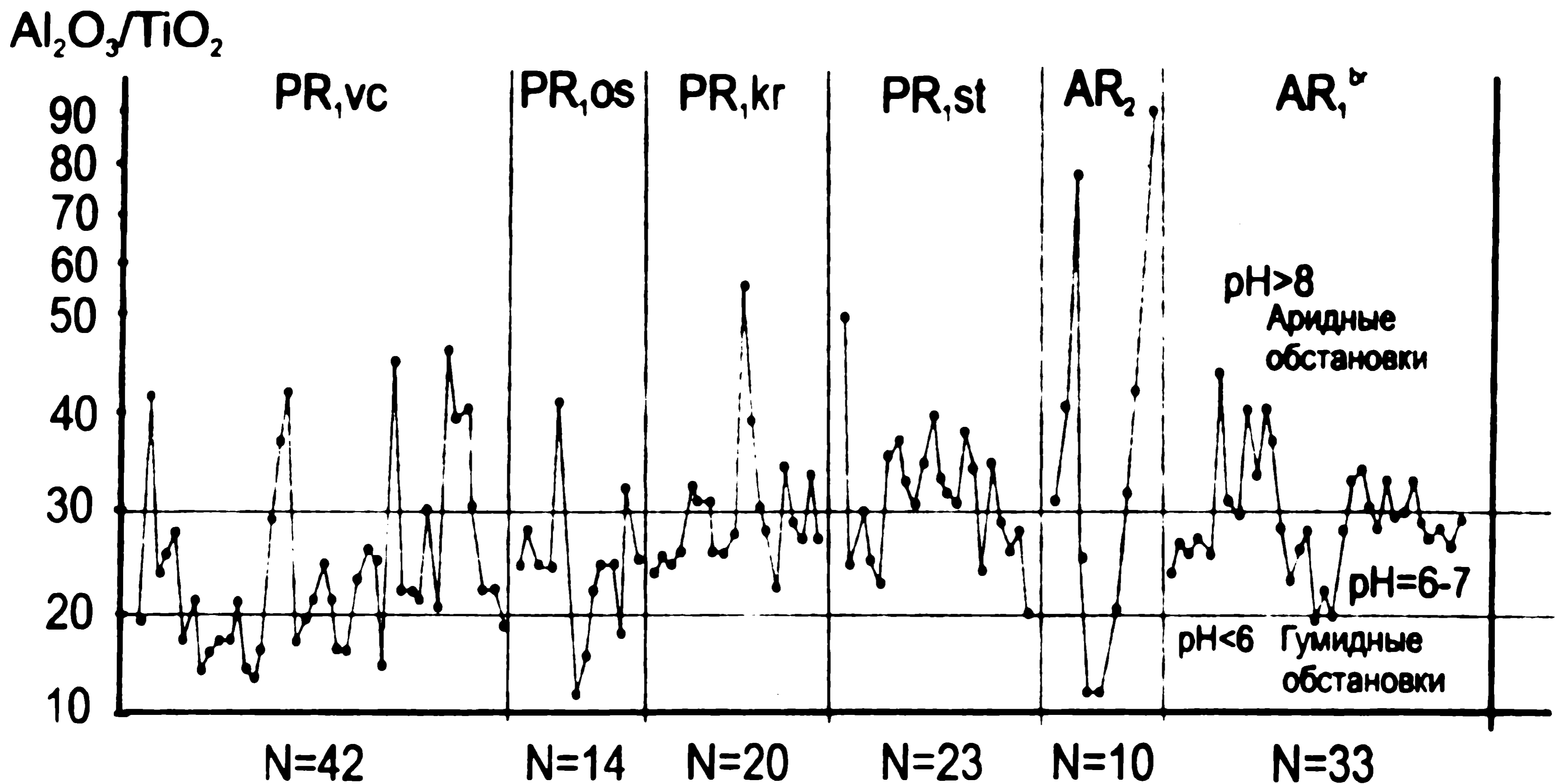
Рис. 2. Вариации значений отношения Al_2O_3/TiO_2 в метапелитах ВКМ
