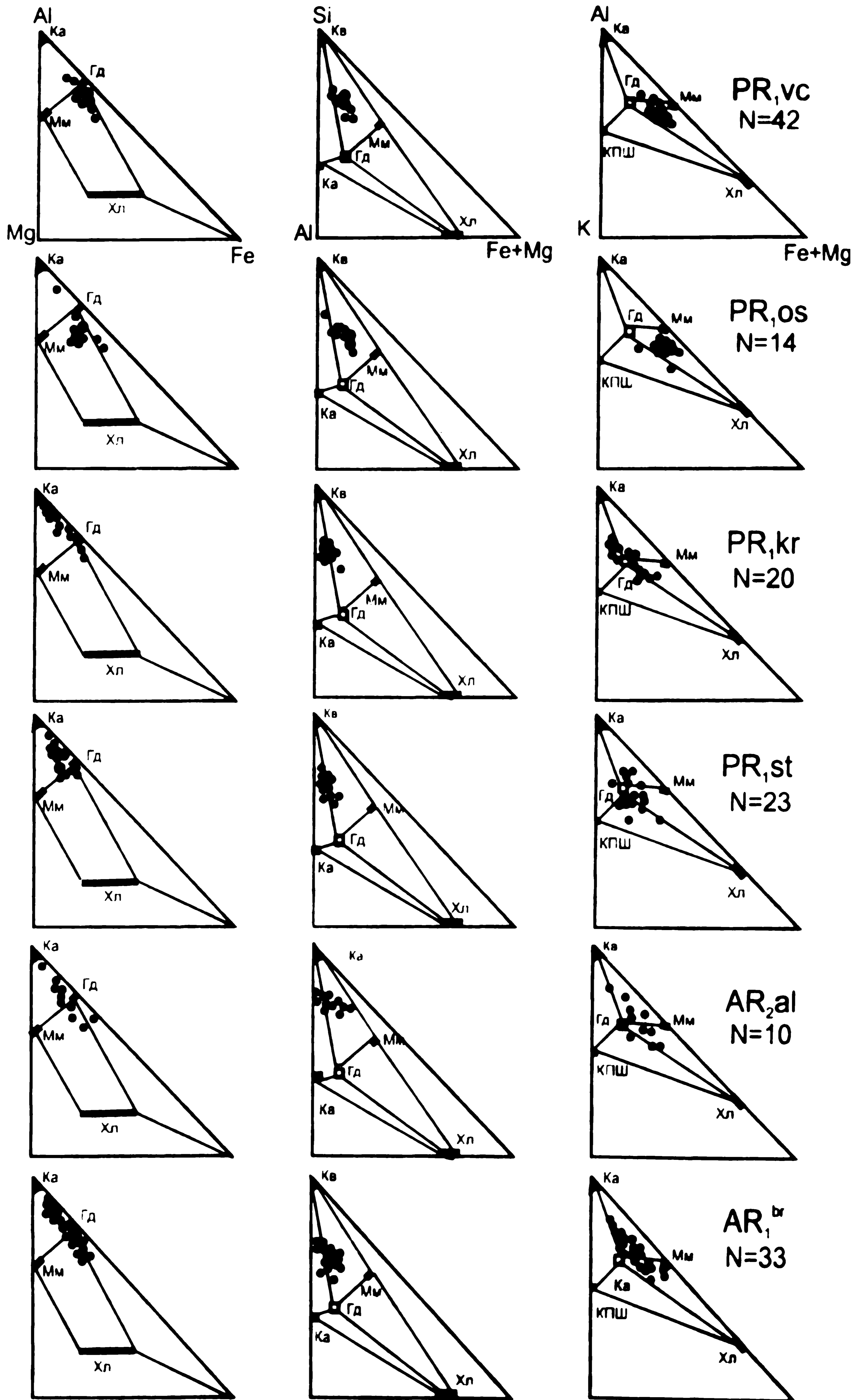
Рис. 1. Проекция составов глиноземистых метапелитов докембрия ВКМ
