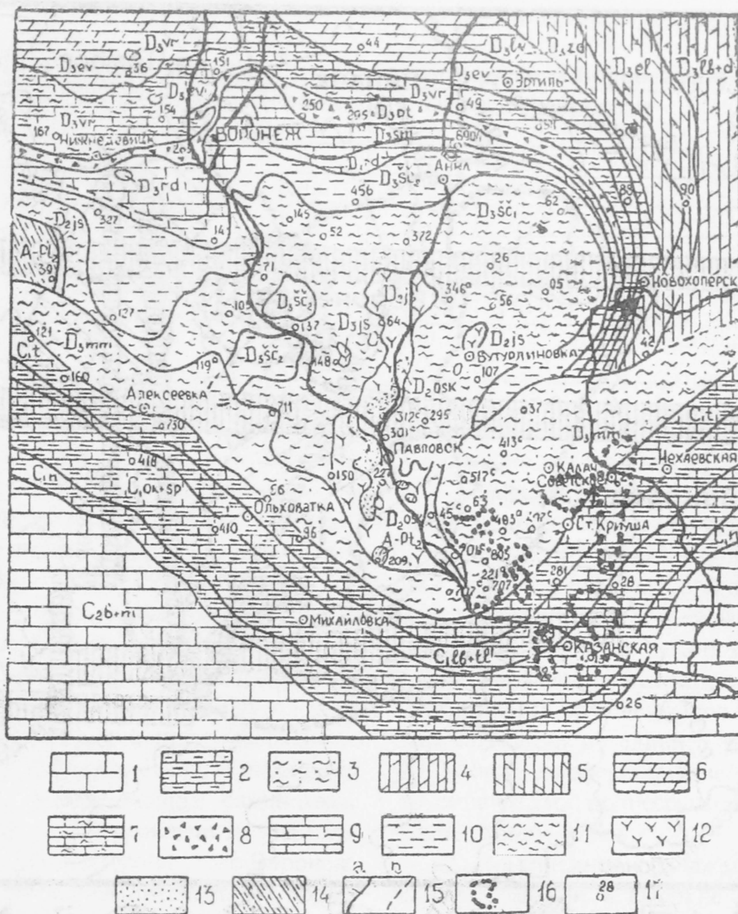
Рис. 1. Геологическая схема домезозойских отложений юго-восточной части Воронежской антеклизы (по В.Ф. Лукьянову, 1970) [14]: 1 - башкирский и московский ярусы нерасчлененные ( C_2b+m ); 2 - намюрский ярус - протвинский горизонт ( C_1n ), визейский ярус - окский и серпуховский надгоризонты нерасчлененные ( C_1ok+sp ), яснополянский надгоризонт - бобриковский и тульский горизонты нерасчлененные ( C_1bb+tl ), турнейский ярус нерасчлененный ( C_1t ); 3 - мамонская толща ( D_3tm ); 4 - лебедянский и данковский горизонты нерасчлененные ( D_3lb+d ); 5 - елецкий горизонт ( D_3el ), задонский горизонт ( D_3zd ); 6 - ливенский горизонт ( D_3lv ), евлановский горизонт ( D_3ev ); 7 - воронежский горизонт ( D_3vor ); 8 - петинский горизонт ( D_3pt ); 9 - семилукский горизонт ( D_3sm ), рудкинский горизонт ( D_3rd ); 10 - верхнешигровский горизонт ( D_3sc_2 ); 11 - нижнешигровский горизонт ( D_3sc_1 ); 12 - ястребовский горизонт ( D_3js ); 13 - староскольский горизонт ( D_2osk ), воробьевский горизонт ( D_2vb ); 14 - архейская и протерозойская группы неразделенные (AR-PR); 15 - геологические границы: а) установленные, б) предполагаемые; 16 - контуры базальтов; 17 - скважины.
