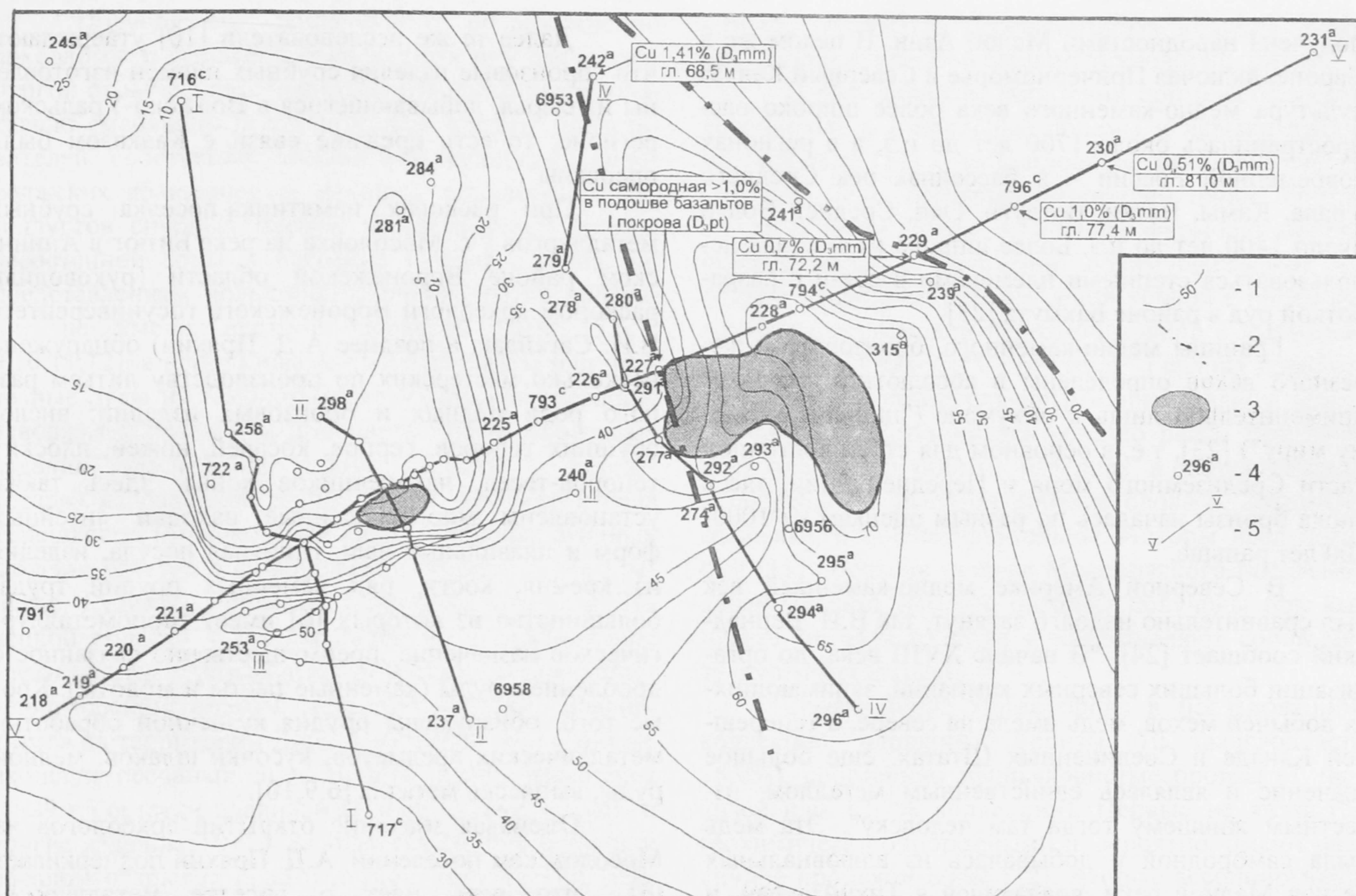
Рис. 7. Схематическая карта мощностей базальтов Подколodновского-Юбилейного лавового поля (по [14]) и выявленные концентрации меди: 1 - изолинии мощностей базальтов; 2 - тектонические нарушения; 3 - жерловая часть вулканической постройки; 4 - скважина и ее номер; 5 - геологические разрезы: I-I, II-II - через Подколodновское месторождение медно-никелевых руд; IV-IV - продольный разрез по Юбилейному месторождению медно-никелевых руд; V-V - вкрест двух месторождений
