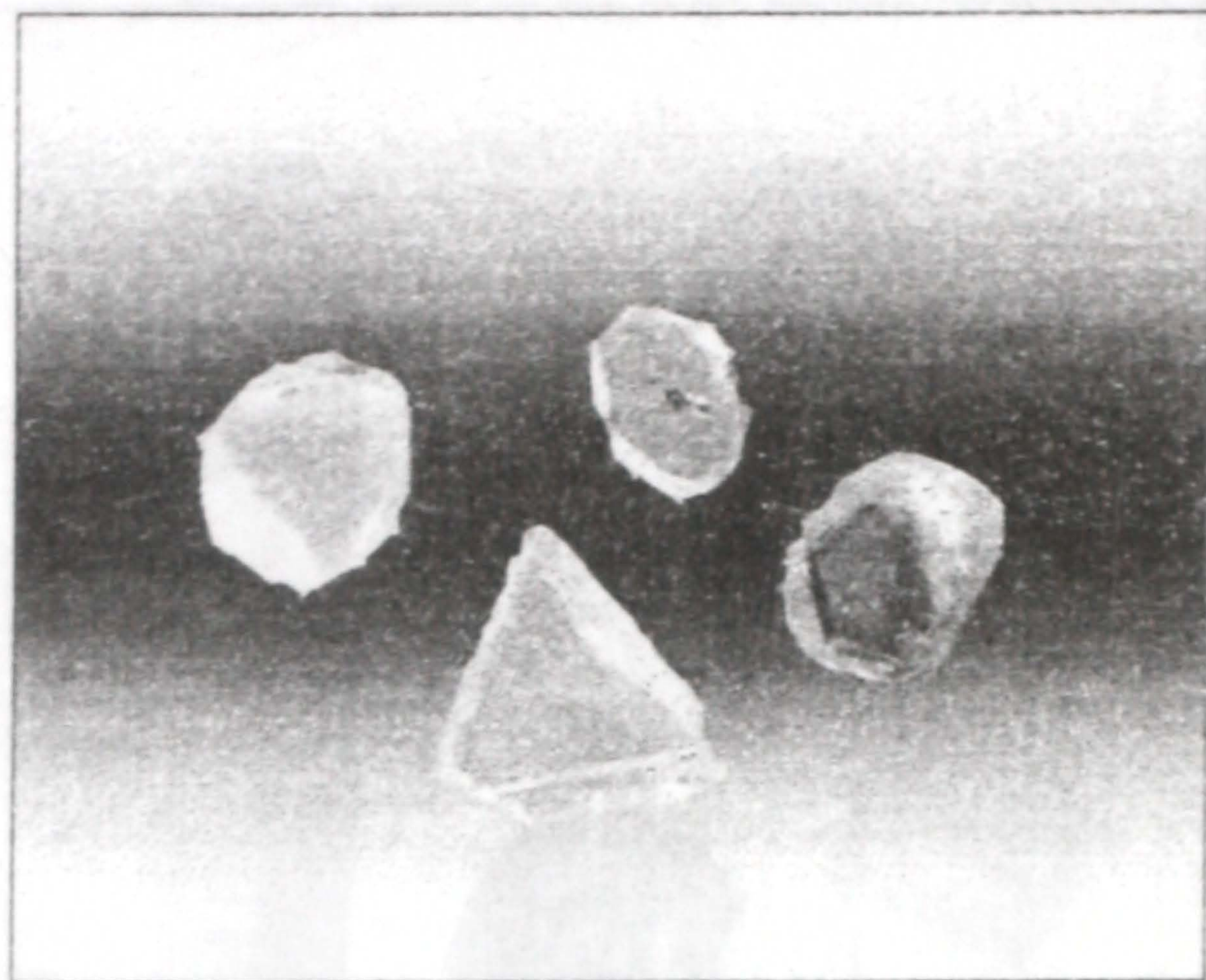
Рис. 11. Алмазы октаэдрического габитуса из россыпей Липецкой области
