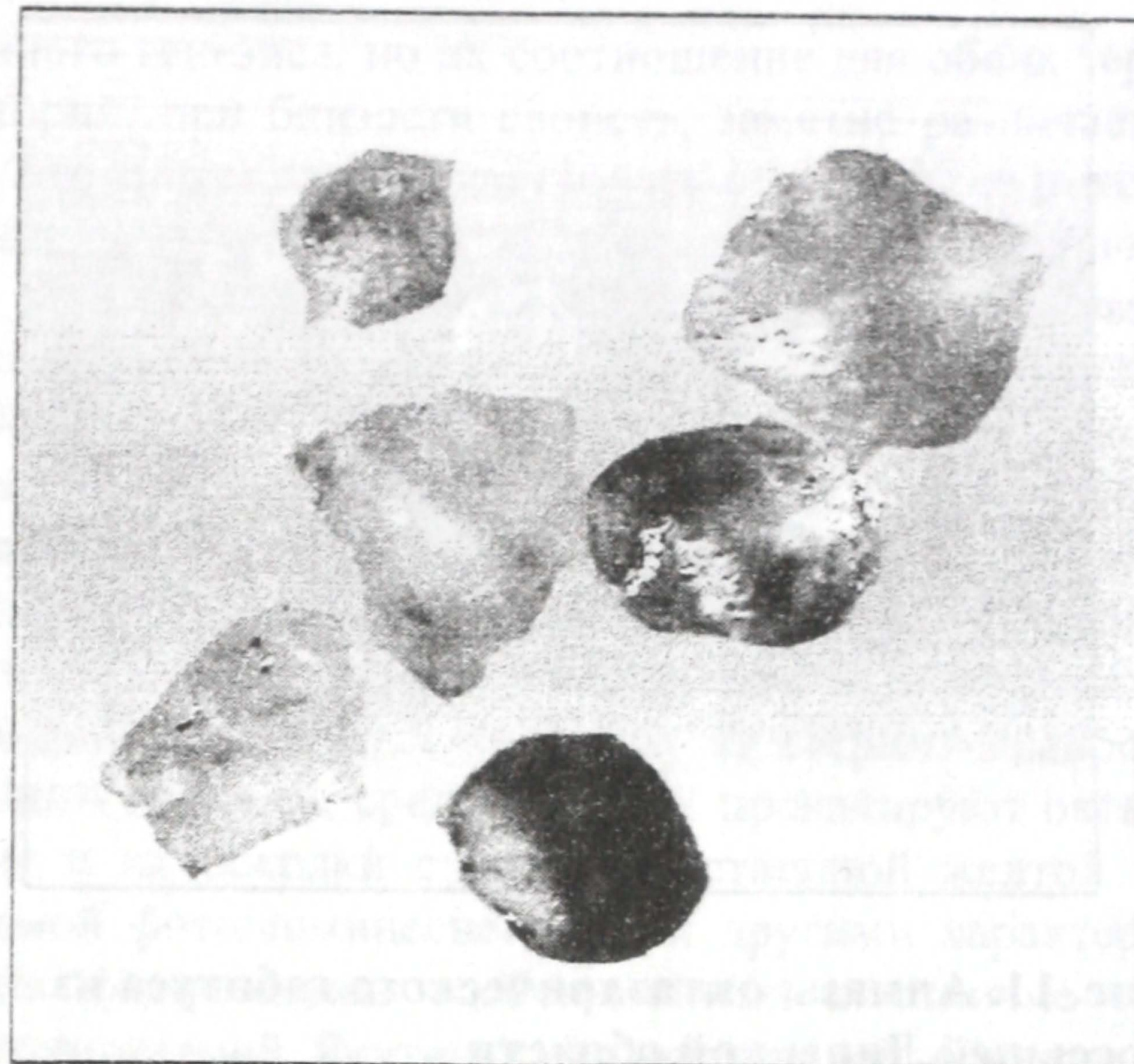
Рис. 10. Общий вид алмазов из россыпей Липецкой области
