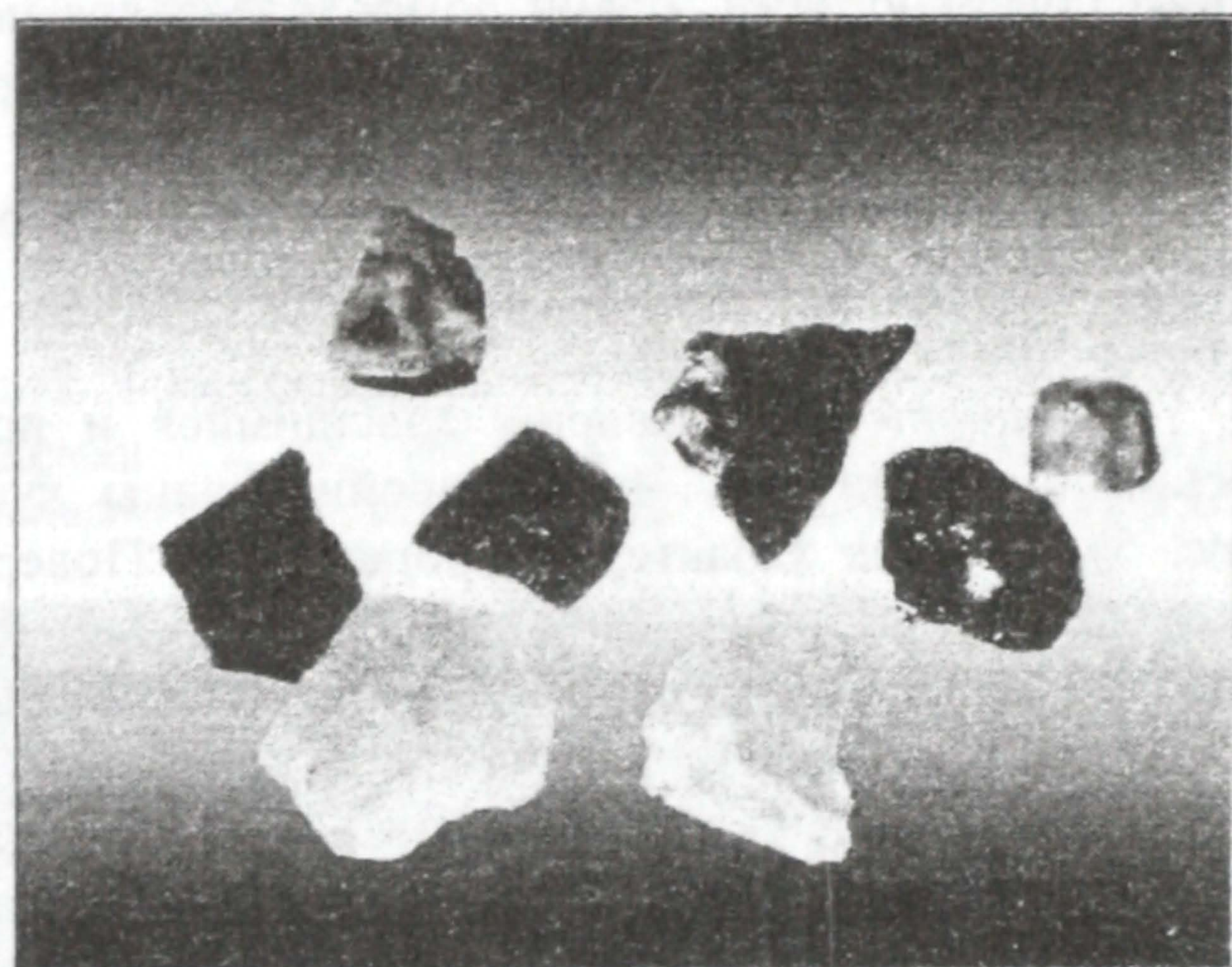
Рис. 7. Алмазы импактного генезиса из россыпей Приднепровья
