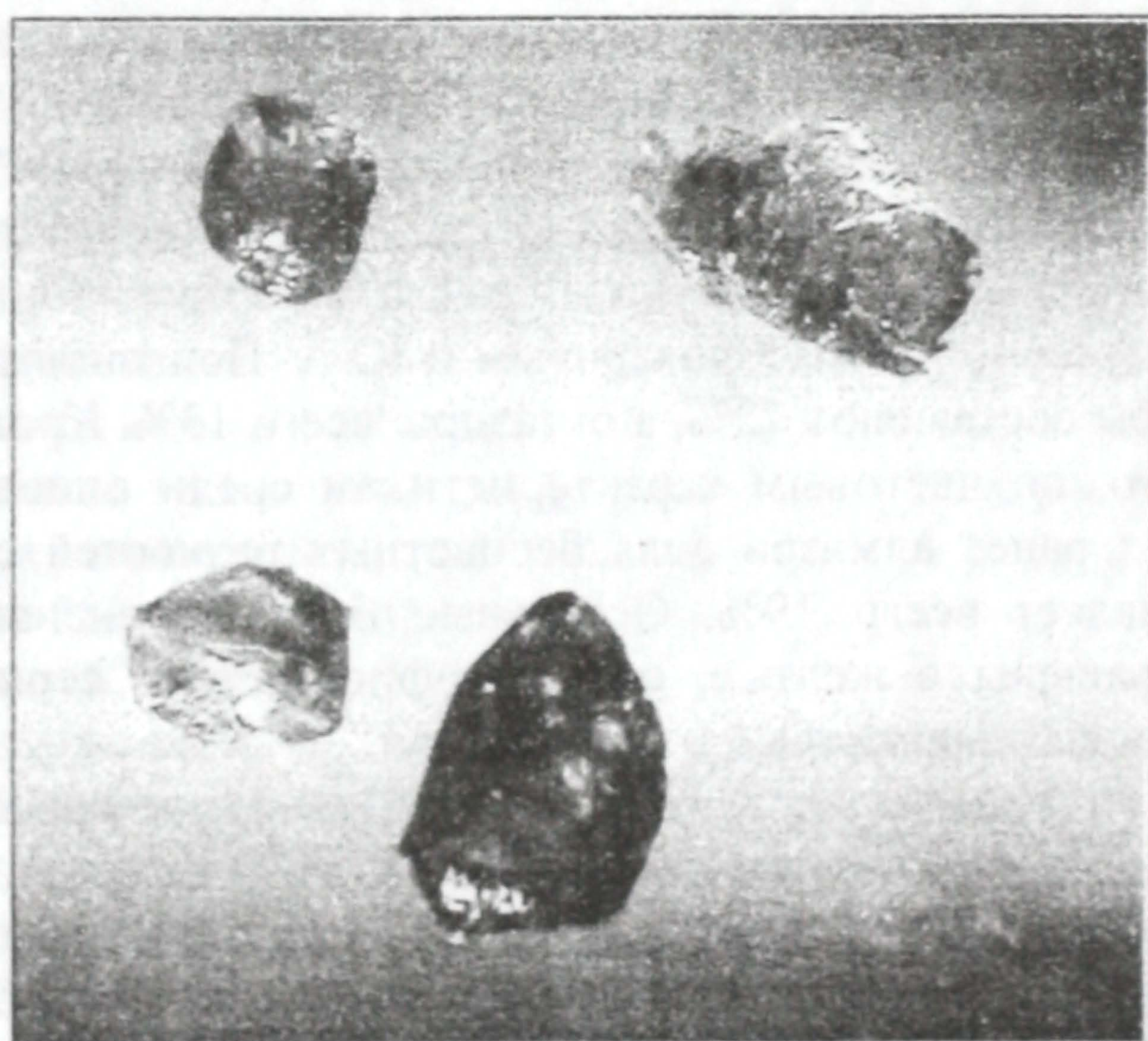
Рис. 13. Алмазы ромбододекаэдрического габитуса из россыпей Липецкой области
