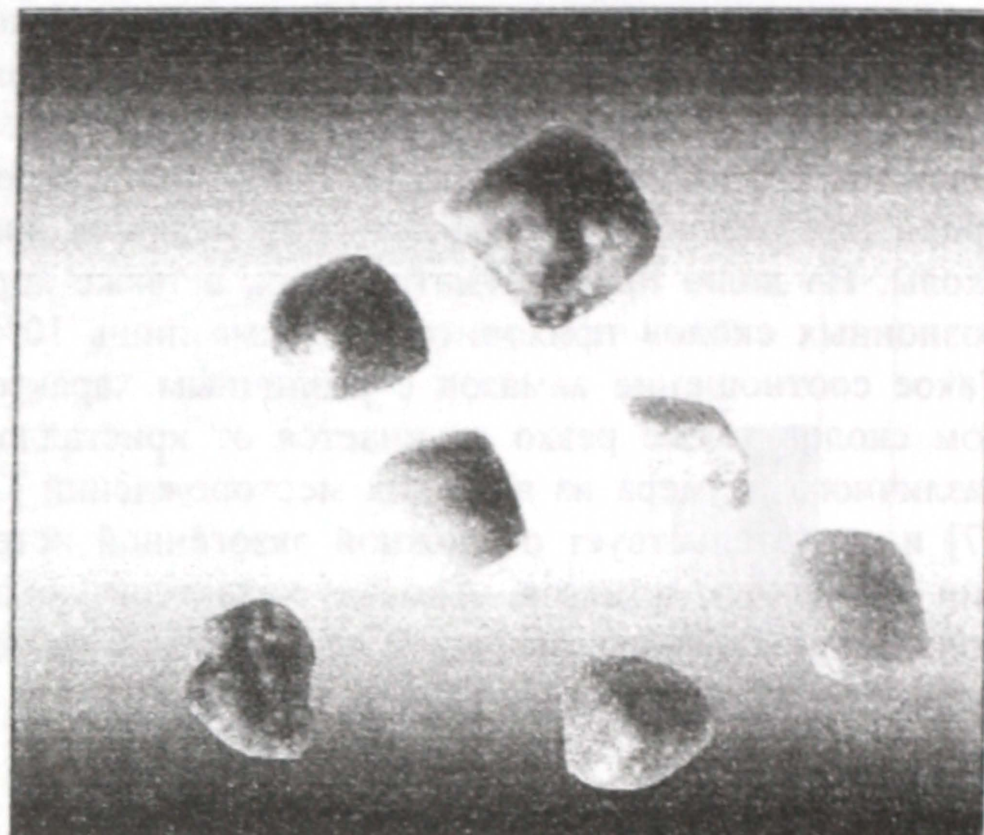
Рис. 14. Карбонадо не выясненного генезиса из россыпей Липецкой области
