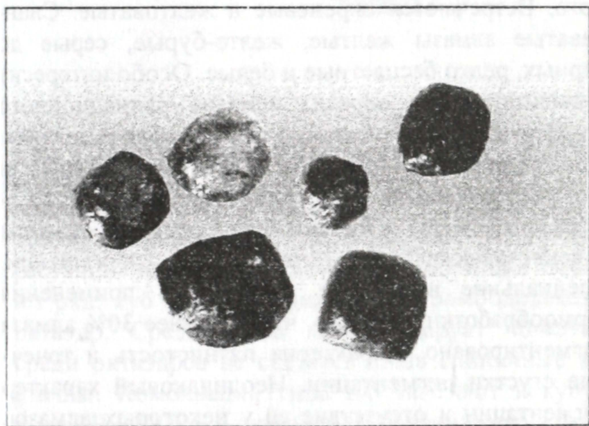
Рис. 5. Алмазы кубического габитуса из россыпей Приднепровья
