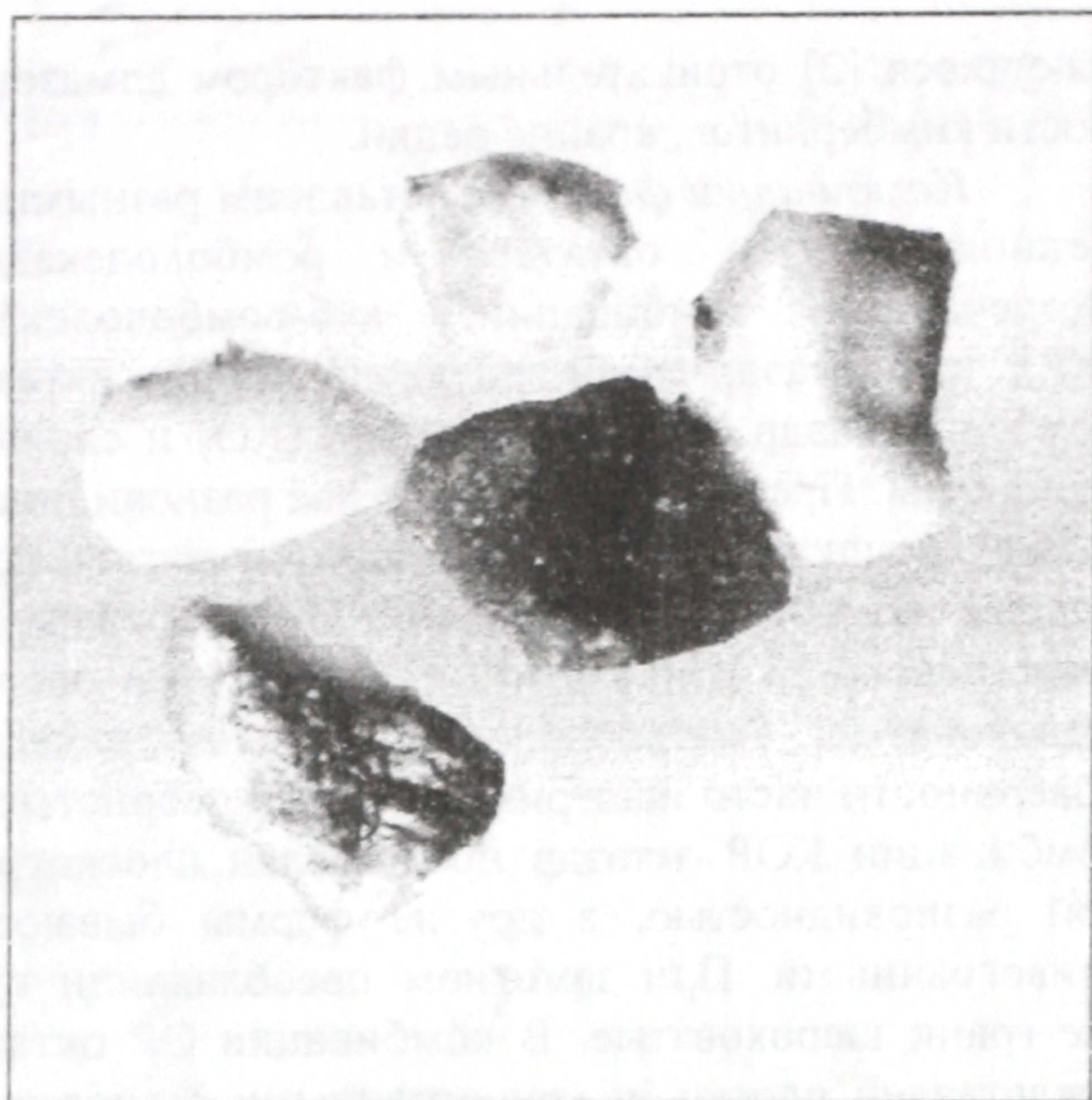
Рис. 6. Карбонадо не выясненного генезиса из россыпей Приднепровья
