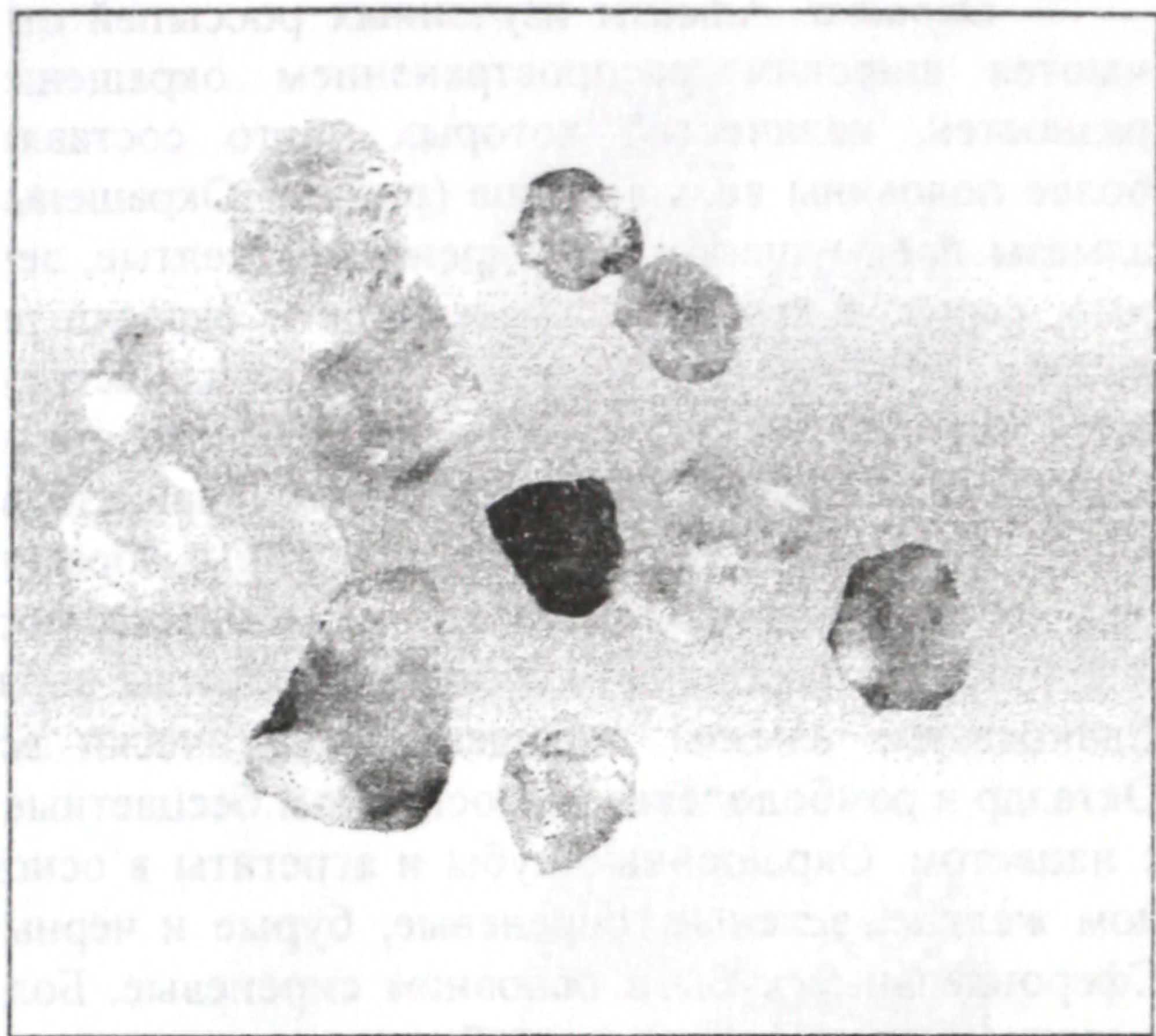
Рис. 4. Алмазы ромбододекаэдрического габитуса из россыпей Приднепровья
