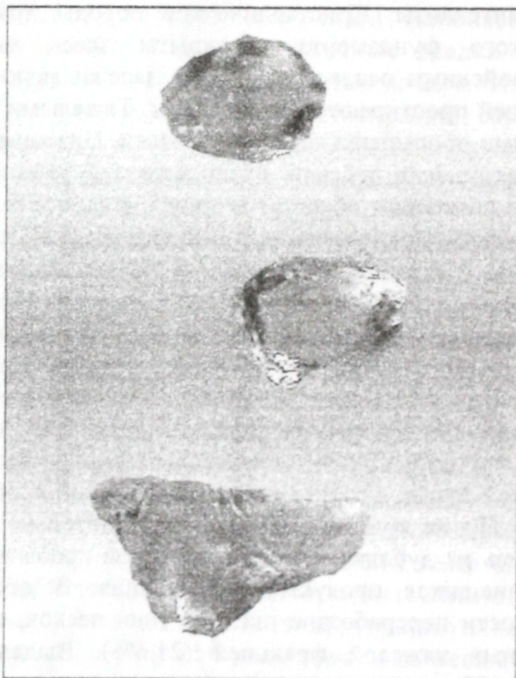
Рис. 3. Алмазы октаэдрического габитуса из россыпей Приднепровья
