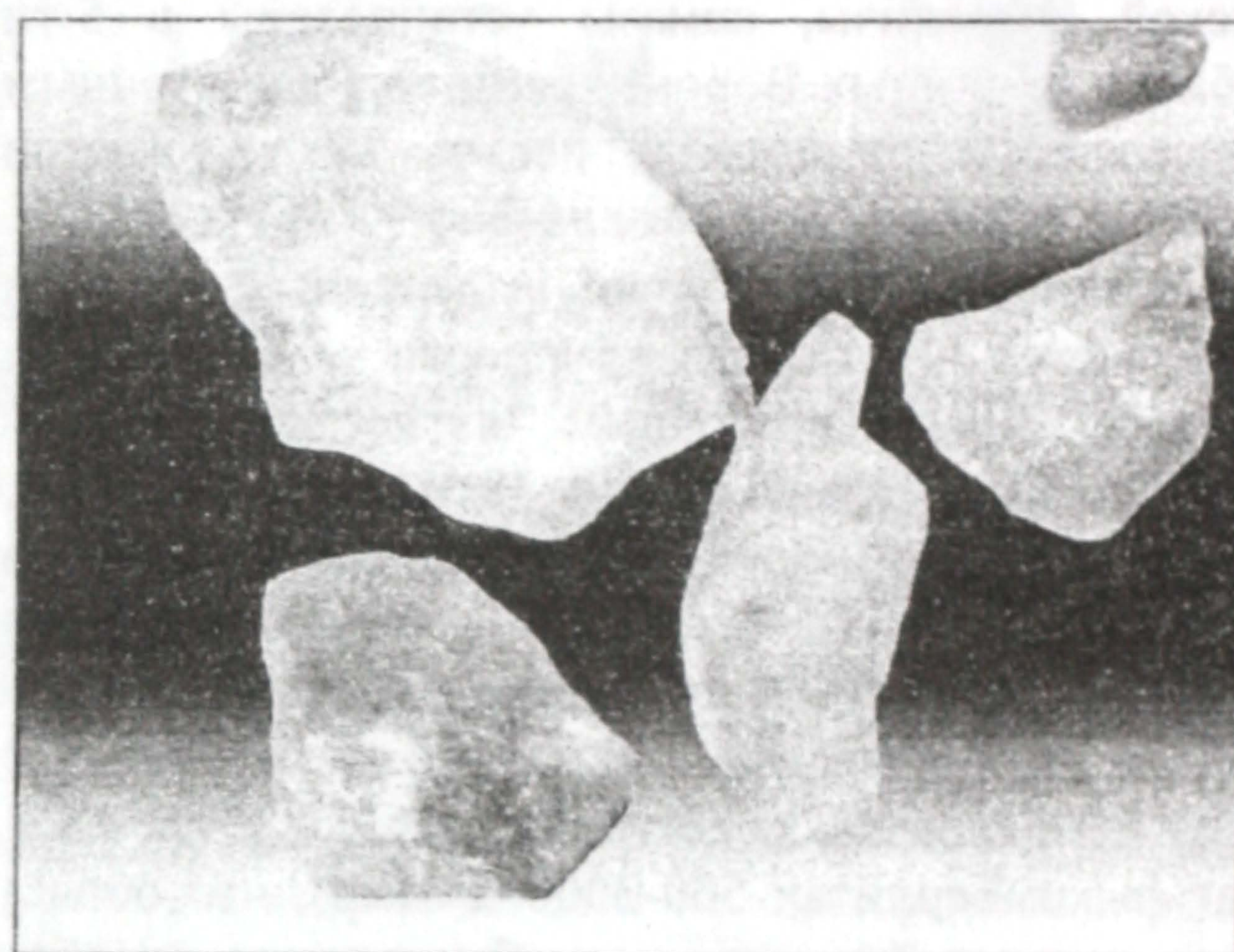
Рис. 15. Алмазы импактного генезиса из россыпей Липецкой области
