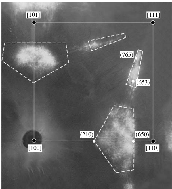
Рис. 3. Фрагмент фотогномограммы кристалла алмаза с участками выпуклых поверхностей додекаэдроиды и тригонгексоктаэдроиды (выделены штриховой линией), принадлежащих симметричным эллипсоидам с одним набором параметров.
