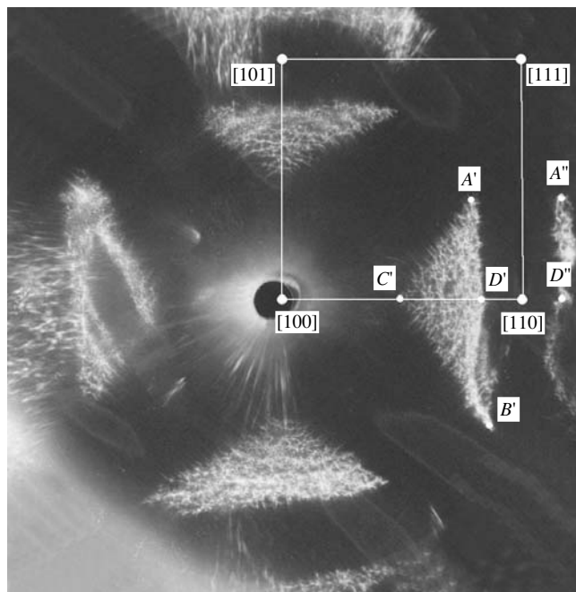
Рис. 1. Фотогномограмма алмаза предельного додекаэдрического типа, ориентированного по оси L^4 , демонстрирующая понижение симметрии формы кристалла до 4/m . Выделены характерные точки рефлекса согласно [6].
