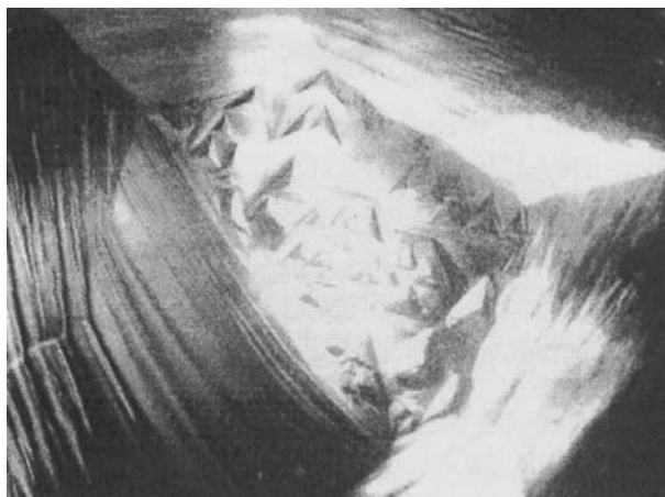
Рис. 4. Поверхность растворенного кристалла алмаза с фрагментами поверхностей реликтовой грани октаэдра, декорированной ямками травления, додекаэдроиды с гранным швом и тригонгексоктаэдроиды, разделенных ребрами.
