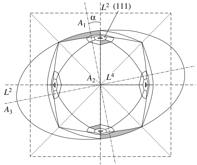
Рис. 2. Эллипсоидная форма округлого кристалла алмаза. Пунктирная линия – исходный октаэдр. Темным цветом отмечены поверхности, принадлежащие выделенному эллипсоиду.
