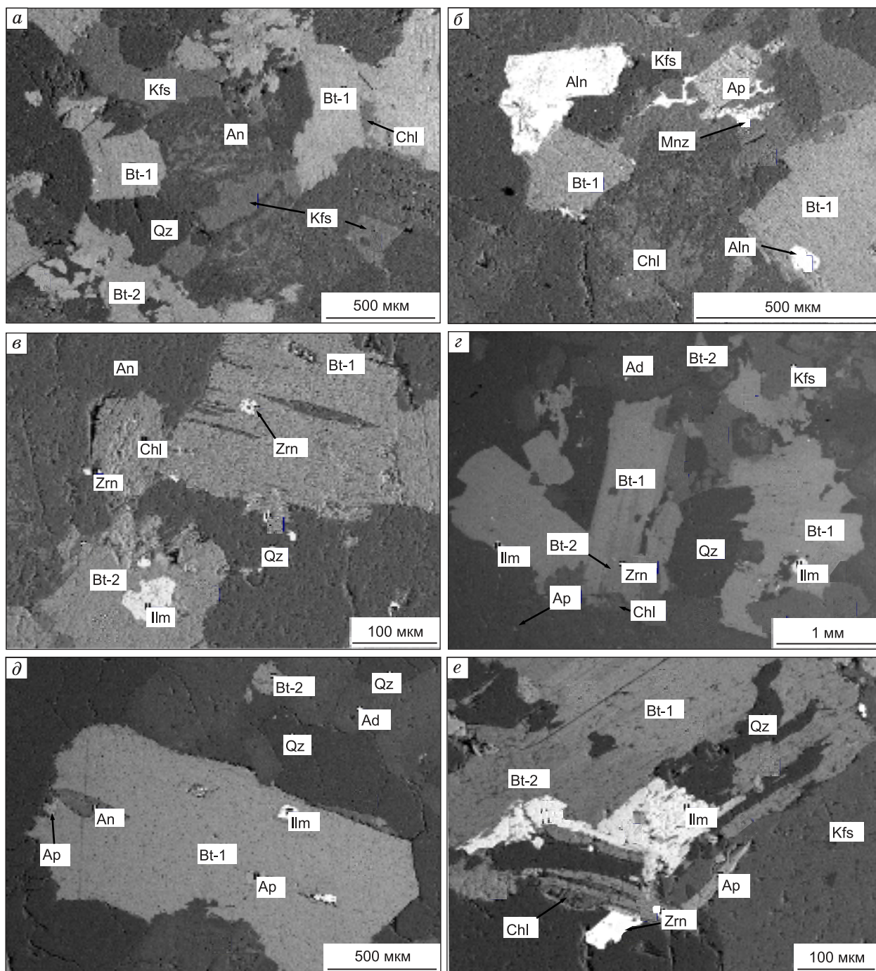
Рис. 5. Микрофотографии шлифов гранодиорита (пр. Б-6) Букесченского (а—в) и гранита (пр. С-3012) Самырского (з—е) массивов.
