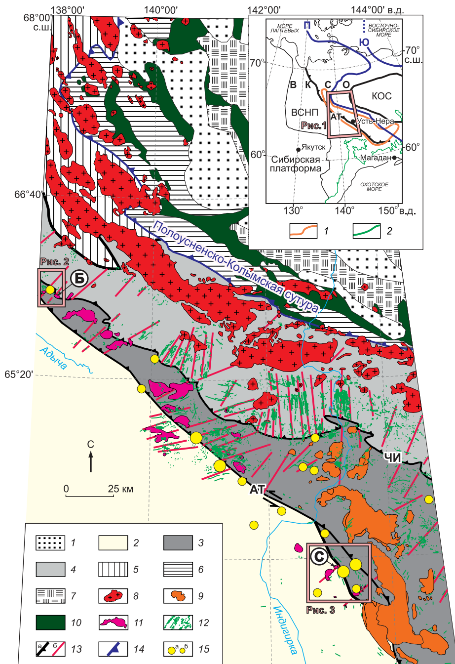
Рис. 1. Схема геологического строения центральной части Верхояно-Колымской складчатой области с исследуемыми объектами, с использованием [Тектоника..., 2001; Toro et al., 2016; Протопопов и др., 2019; Fridovsky et al., 2020].
