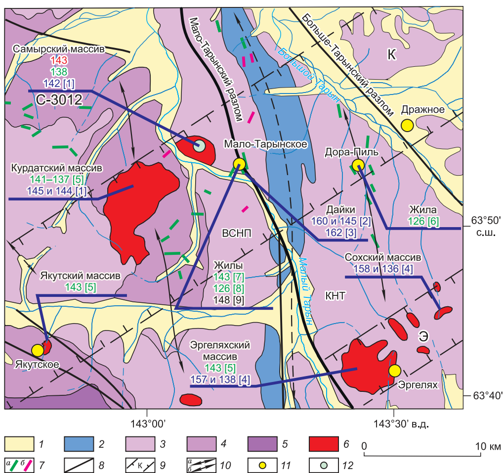
Рис. 3. Схема геологического строения с проявлениями гранитоидов комплекса малых интрузий района междуречья Малого Тарына и Большого Тарына, с использованием [Зайцев и др., 2017].
