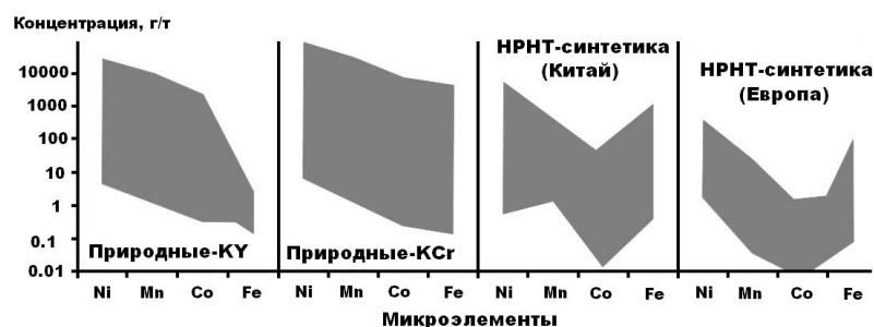
Рис. 6. Сопоставление алмазов из тибетских офиолитов и синтетических аналогов по содержанию примесей металлов группы железа
