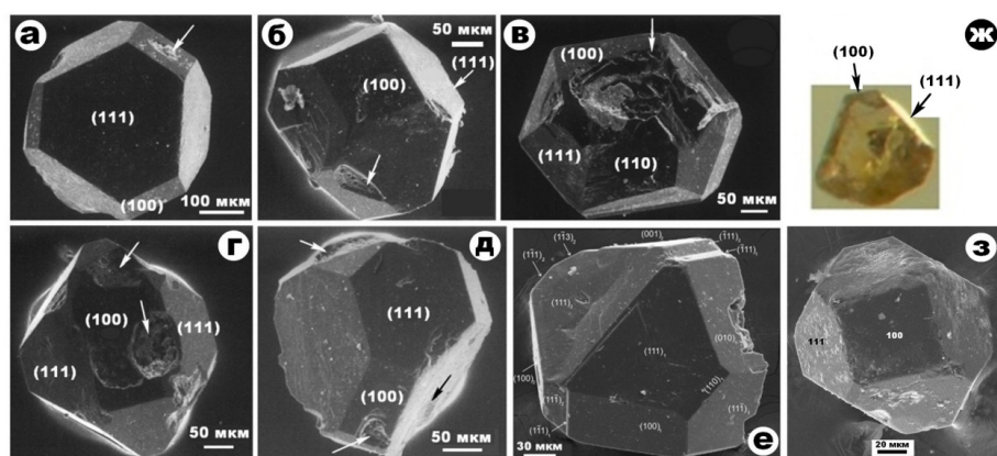
Рис. 3. Кристалломорфология толбачинских алмазов: а–ж – из продуктов ТТИ-50, з – из продуктов БТТИ или более ранних извержений. Фото- (ж) и СЭМ-изображения в режиме вторичных электронов (а–е, з)
