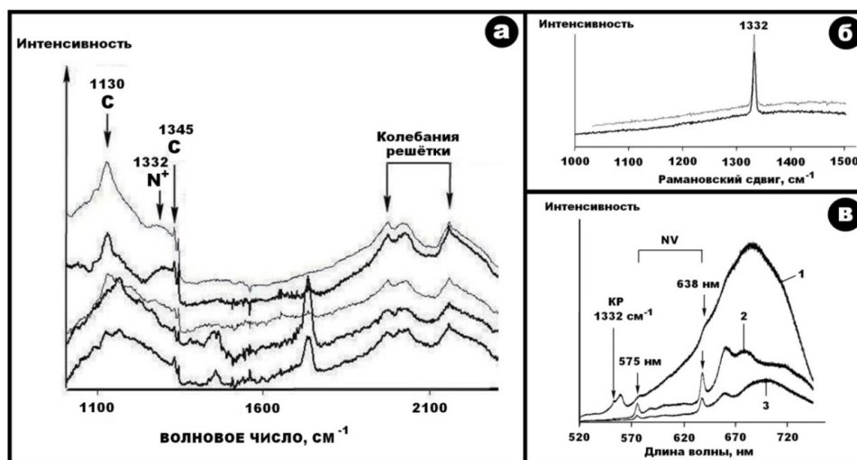
Рис. 7. Спектроскопические свойства и состояние азотных дефектов в толбачинских и ключевских алмазах: а – спектры ИК поглощения, б – спектр КР, в – спектры КР и люминесценции
