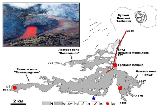
Рис. 1. Карта продуктов ТТИ-50 (показаны серым цветом): 1 – лавовое поле начального периода извержения; 2 – лавовые поля более позднего периода извержения; 3 – абсолютные отметки высот; 4 – старые трещины; 5 – трещины, через которые происходило извержение; 6 – алмазоносные участки лавовых потоков ТТИ-50. Синей звездочкой отмечено место находки алмазов в продуктах более ранних извержений, отстоящее к югу от ТТИ-50 на 10–12 км
