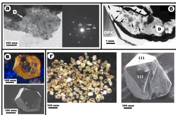
Рис. 2. Примеры природных некимберлитовых алмазов: а – из современных пеплов вулкана Эйяфьядлайёкюдль, Исландия; б – из гавайских океанических базальтоидов – стрелками показаны облакоподобные сгущения наноалмазов, D – индивид микрометровой размерности; в – алмазы из офиолитов массива Луобуза, Тибет; г – алмазы из офиолитовых хромититов массива Рай-Из, Полярный Урал, Россия
