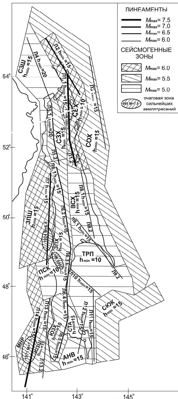
Рис. 3. Конфигурация и параметры зон источников в линейментно-доменной модели ИМГиГ-97 (по Л.С. Оскорбину [3]).
