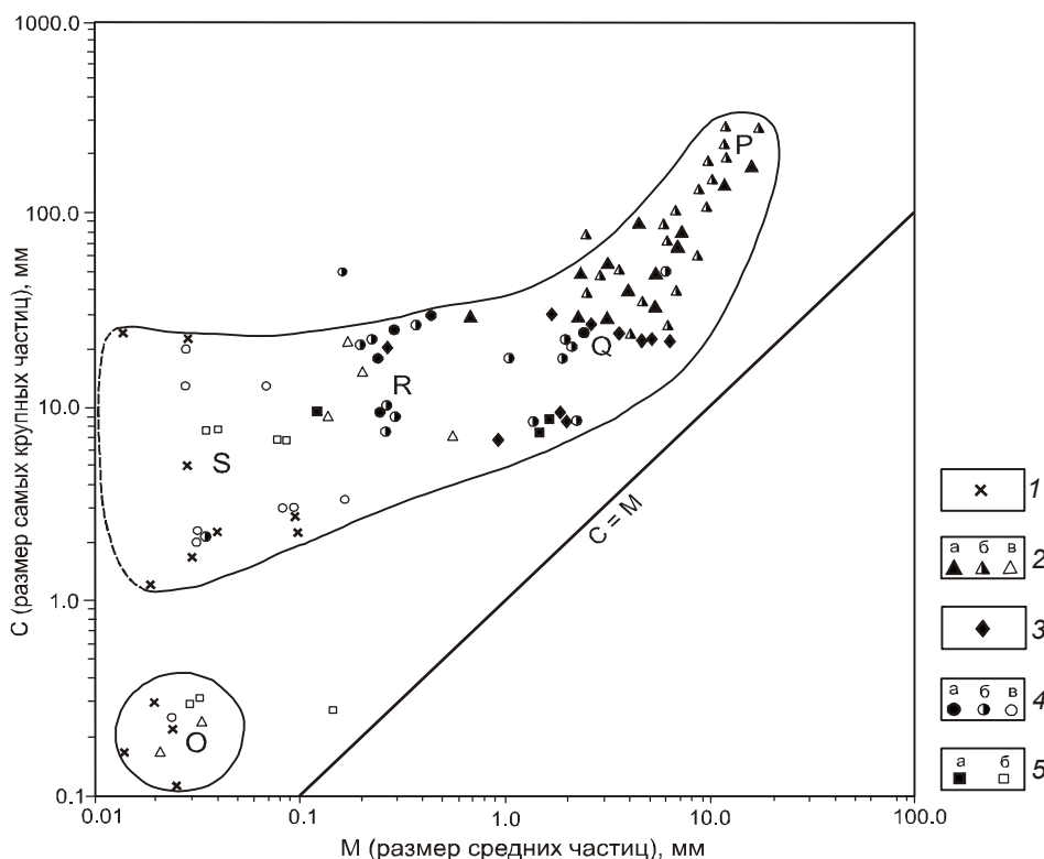
Рис. 5. График распределения максимальных (С) и медианных (М) размеров частиц в рыхлых отложениях в Анойской впадине и речных долинах на ее окраине.
