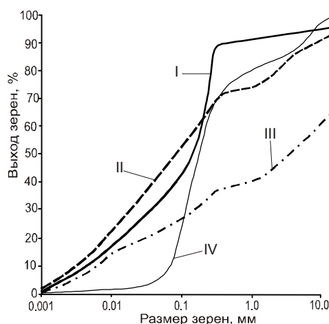
Рис. 4. Кумулятивные кривые отложений покровного ледового комплекса (I), реликтовых частей коры выветривания (II), элювиальных образований (III) и пойменной фации аллювия (IV) в долине р. Тополевка.
