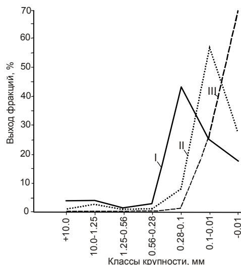
Рис. 3. Графики гранулометрического состава отложений покровного ледового комплекса в речных долинах в пределах переходной зоны (I), периферийных (II) и центральных (III) частях Анюйской впадины.
