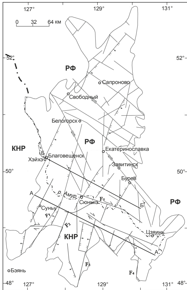
Рис. 2. Схема размещения основных разломов в Суньцзянь-Цзяньцзяньском и Зейско-Буреинском бассейнах. По материалам Дацинской нефтяной компании, Г.А. Шаткову и др. [22], А.П. Сорокину и Т.В. Артеменко [27].
