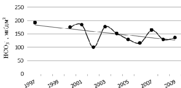
Рис. 3. Динамика среднегодовых концентраций иона \text{HCO}_3^- в водах р. Икса – с. Плотниково
