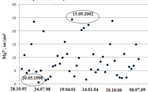
Рис. 1. Распределение проб с концентрациями ионов магния в водах р. Андарма – с. Панычево (в хронологическом порядке)
