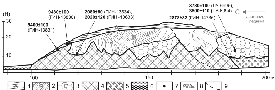
Рис. 2. Геологическое строение напорного вала ледника Грэнфиордбреен
