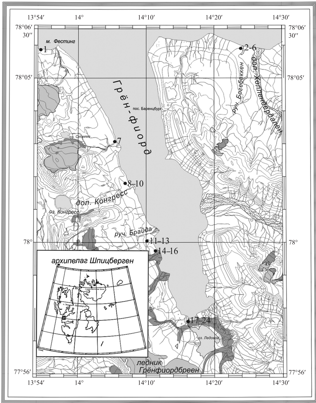
Рис. 1. Места отбора проб на радиоуглеродный анализ. Масштаб 1:200000. Номера соответствуют порядковым номерам проб (см. табл.)
