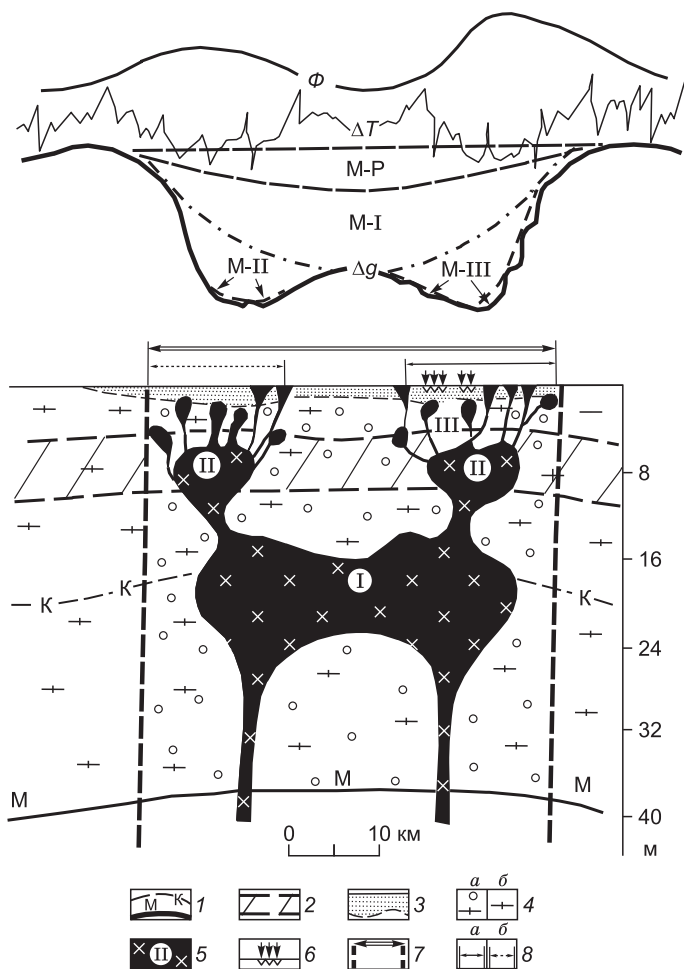
Рис. 5. Генерализованный геолого-геофизический разрез Алданского золоторудного района, по [Абрамов, 1995] с некоторыми изменениями.
