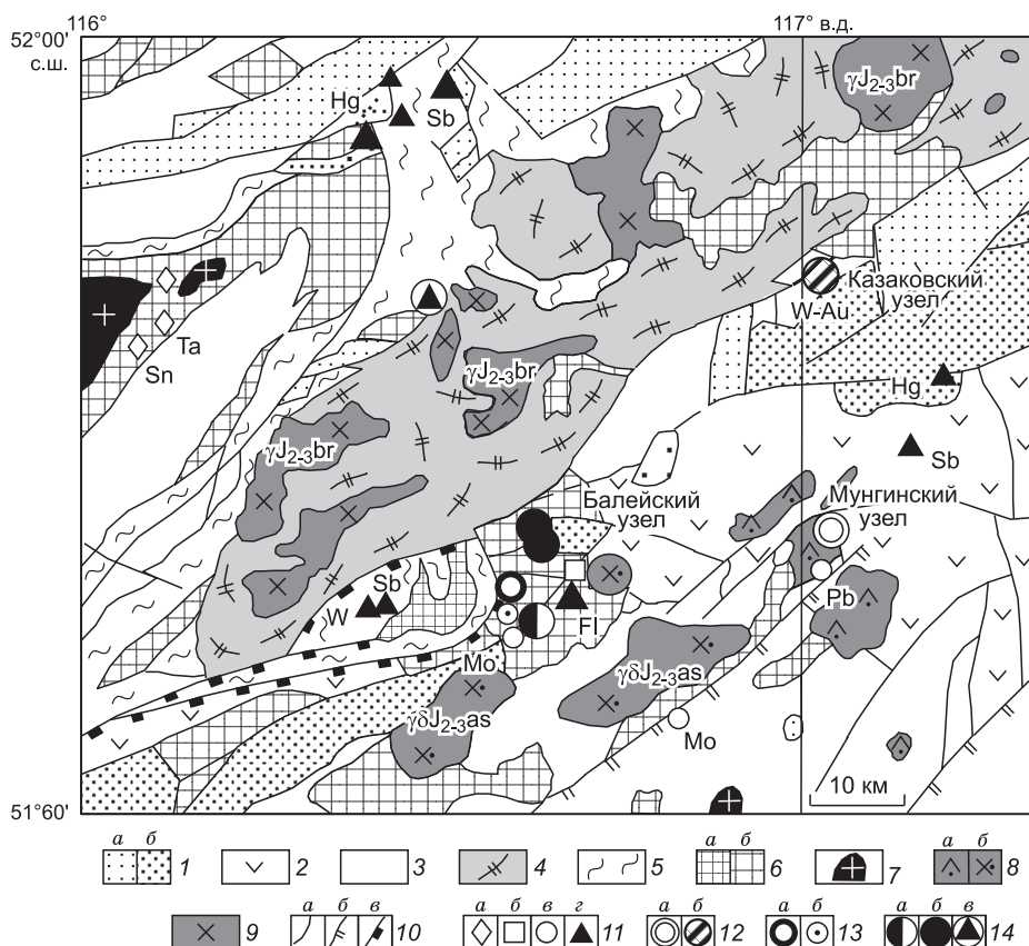
Рис. 6. Схематическая геолого-металлогеническая карта БалеЙского рудного района (Забайкалье), по [БалеЙское..., 1984; Карта..., 2005] с некоторыми изменениями.
