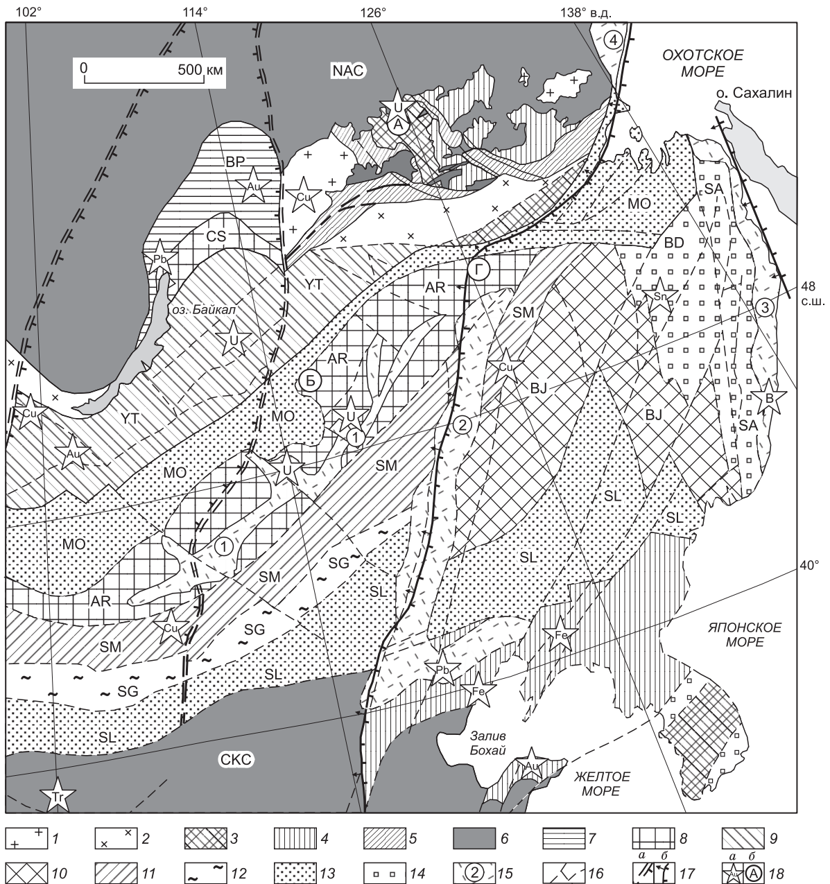
Рис. 3. Схема тектонического районирования Центрально-Азиатского пояса и прилегающих кратонов (древних платформ), по [Тектоника..., 2001, 2004; Парфенов и др., 2003] с некоторыми изменениями и дополнениями.
