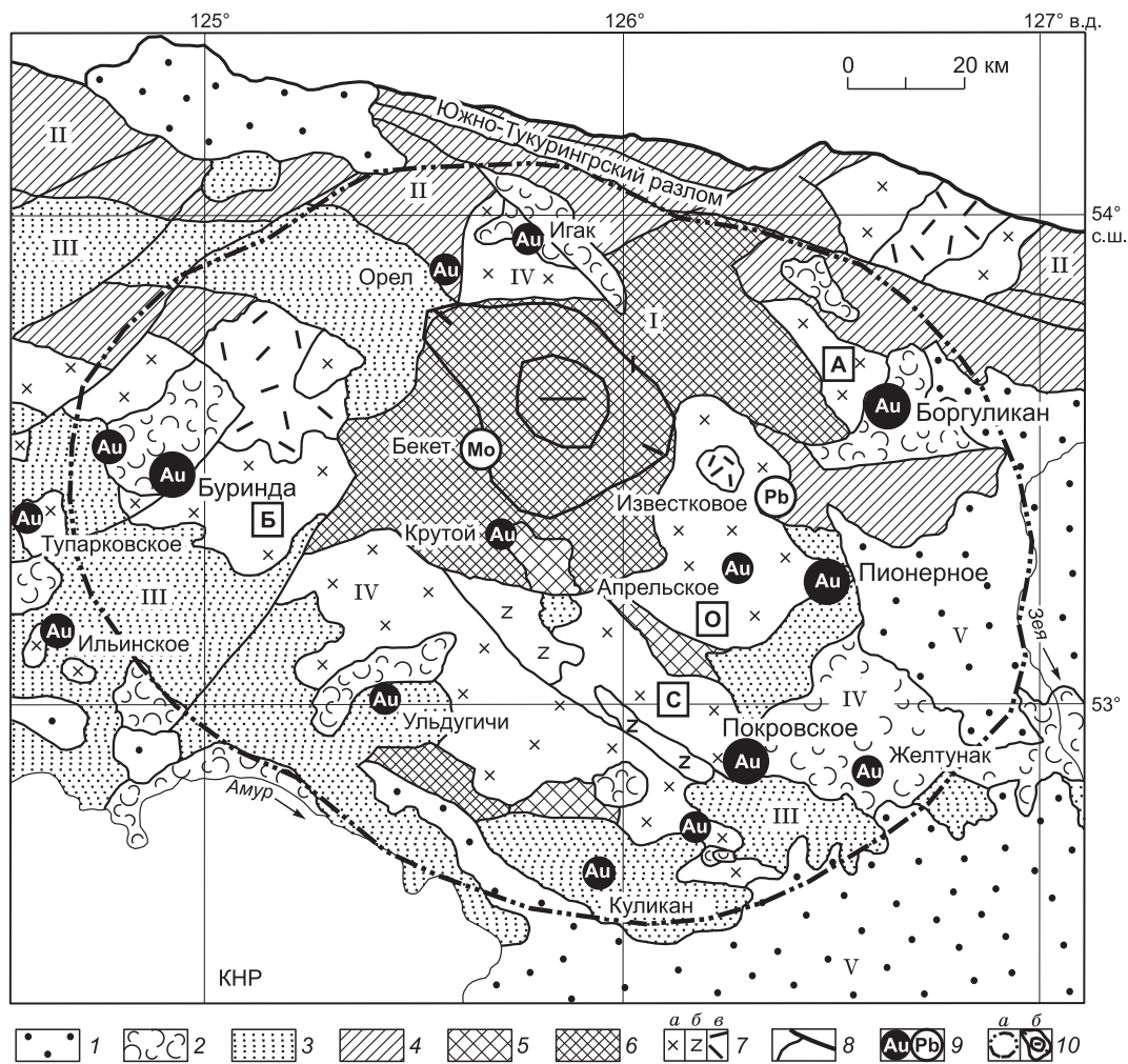
Рис. 7. Структурно-металлогеническая схема Гонжинского рудного района (Верхнее Приамурье).
