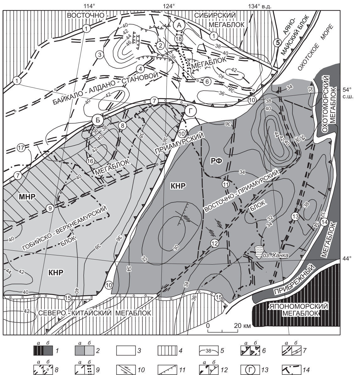
Рис. 1. Схема глубинного строения Приамурья и сопредельных регионов (на основе районирования гравитационного поля), по [Тектоника..., 2004; Хомич, Борискина, 2007] с некоторыми изменениями и дополнениями.
