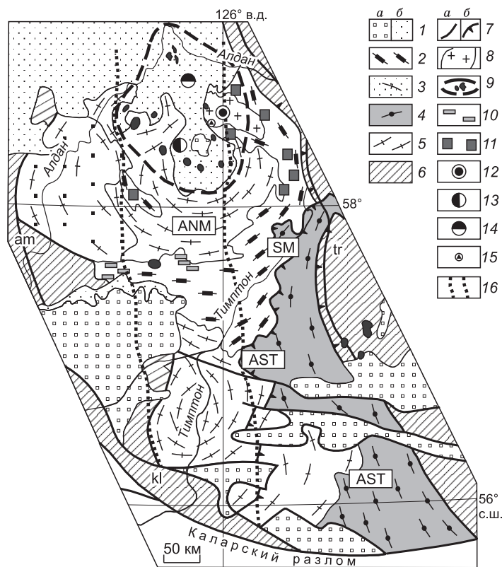
Рис. 4. Схематическая геолого-металлогеническая карта Центрально-Алданского супертеррейна, по [Тектоника..., 2001; Казанский, 2004] с изменениями.
