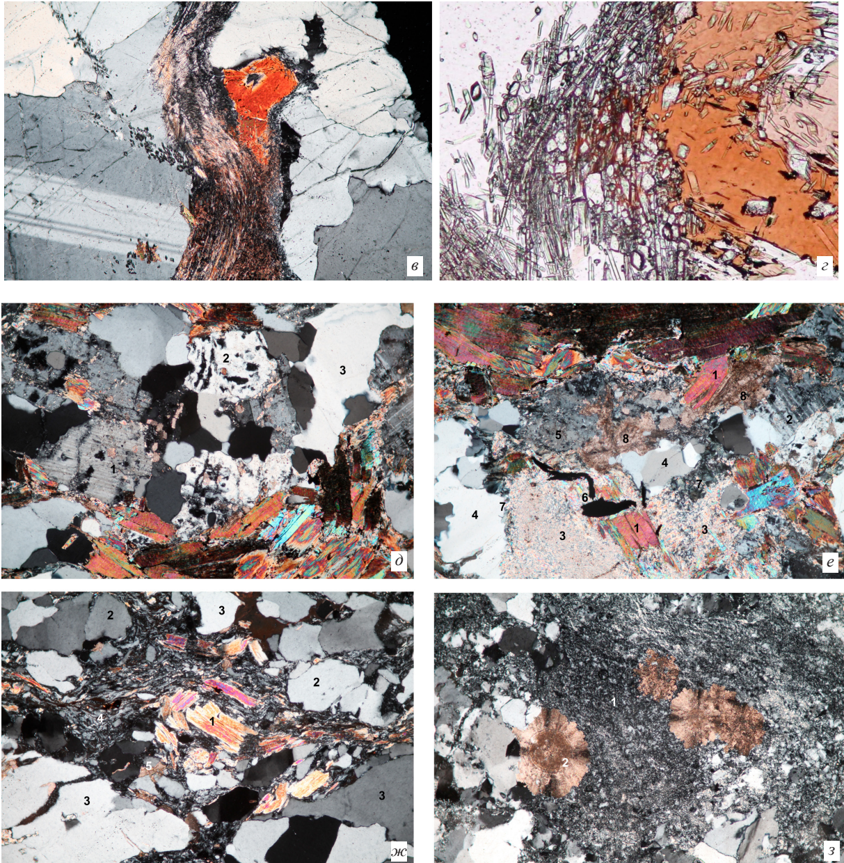
Продолжение. Петрографические шлифы керн скважин Пальяновской площади: б – гранит биотитовый. Спиралевидная структура струйно-поточкового образования. Скв.153. Шлиф 15-5а. Глубина 2687,5м. С анализатором. Увел. 100х; з – диссоциация биотита и формирование амфибол-скаполитовой ассоциации струйно-поточкового образования. Гранит биотитовый. Скв. 153. Шлиф 15/6. Без анализатора. Увел. 400х; д – гранит биотитовый в начальной стадии гидротермального изменения. «Дырчатая» калишпатизация (1) и окварцевание плагиоклаза (2) и разрастание кварца (3). Скв.138. Шлиф 22/1а. Глубина 2859,9 м. С анализатором. Увел 100х; е – гранит биотитовый, гидротермально измененный, с реликтами биотита (1) и плагиоклаза (2) и новообразованиями серицита (3), кварца (4) и калишпата (5), сульфидами (6), селадонитом (7) и карбонатом (8), окрашенным битумом. Скв.138. Шлиф 21. Глубина 2851,8 м. С анализатором. Увел 100х; ж – катаклазит по гранитоиду. Биотит (1), ортоклаз (2) и кварц (3). Зонки серицит-кварцевого состава (4) с кальцитом (5). Скв. 600. Шлиф 17. Глубина 2427,5м. С анализатором. Увел 100х; з – катаклазит по гранитоиду, гидротермально переработанный. В центре зонка серицит-калишпат-кварцевого состава (1) и сферокристаллы сидерита (2). Скв. 611. Шлиф 25–2 Глубина 2418,7м. С анализатором. Увел 100х
