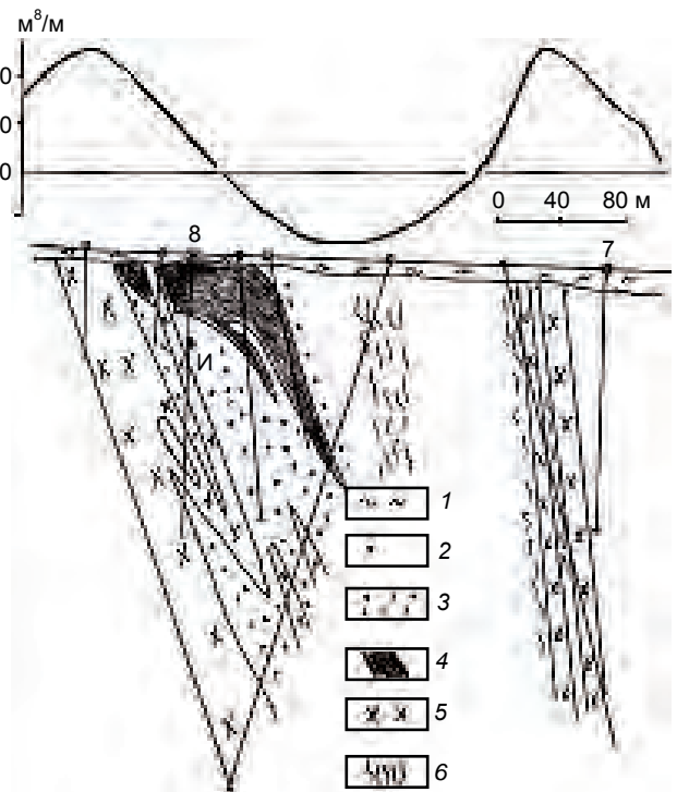
Рисунок 6. Пример проявления малых интрузий в форме даек, которые отметились положительными аномалиями градиента потенциала поля погруженного источника тока, на одном из разведочных профилей с соответствующим геологическим разрезом. 1 – покровные отложения; 2 – вулканогенные породы; 3 – сульфидизация пород; 4 – руды; 5 – габбро-диоритовые тела даек; 6 – зоны трещиноватости и рассланцевания; И – точечный источник тока (по материалам Уральской геолого-съемочной экспедиции, Р. Ф. Гилаздинова, В. М. Сапожникова) / Figure 6. An example of manifestations of small intrusions in the form of dikes, which were noted with the positive anomalies of the field potential gradient of immersed current source, in one of the exploratory profiles with the corresponding geological section (based on the Ural geological survey expedition and R. F. Gilazdinov, V. M. Sapozhnikov).
