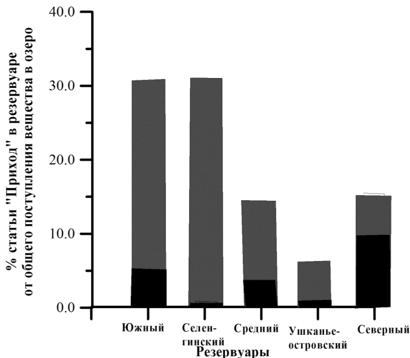
Рис. 4. Внешние и внутренние нагрузки на протяжении озера Байкал (статья «Приход»)
