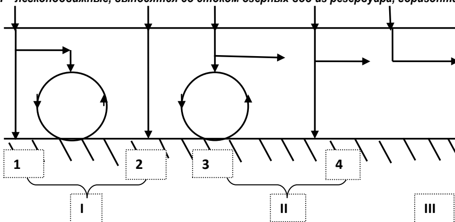
Рис. 2. Пространственная миграция компонентов в водах Селенгинского резервуара: I – слабоподвижные компоненты, находящиеся в водах резервуара в основном в виде взвеси, накапливаются: 1 – в донных отложениях и в водах, часть вещества переходит из твердой фазы в раствор (находится в водах резервуара в виде взвеси и в виде растворенного вещества) и участвует в химических круговоротах; 2 – в донных отложениях; II – умеренно подвижные, находятся в твердой и растворенной формах, частично выносятся со стоком озерных вод из резервуара, частично накапливаются: 3 – в водах и донных отложениях, участвуют в химических круговоротах; 4 – в донных отложениях; III – легкоподвижные, выносятся со стоком озерных вод из резервуара, в резервуаре находятся в растворенной форме
