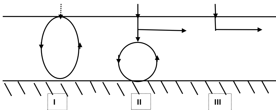
Рис. 3. Пространственная миграция компонентов в водах Северного резервуара: I – слабоподвижные компоненты, находятся в твердой и растворенной формах, передвижение «вниз-вверх» в пределах резервуара, связываются и накапливаются в донных отложениях и в водах, участвуют в химических круговоротах; II – умеренно подвижные, находятся в твердой и растворенной формах, частично выносятся со стоком озерных вод из резервуара (частичная горизонтальная миграция), остальная часть связывается и накапливается в донных отложениях и в водах, участвует в химических круговоротах (передвижение «вниз-вверх»); III – легкоподвижные, в резервуаре находятся в растворенной форме, выносятся со стоком озерных вод из резервуара, горизонтальная миграция
