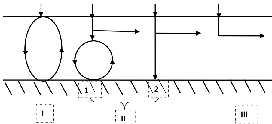
Рис. 1. Пространственная миграция компонентов в водах Южного, Среднего, Ушканьеостровского резервуаров: I – слабоподвижные компоненты, вертикальная миграция, накапливаются в донных отложениях и в водах, участвуют в химических круговоротах; II – умеренно подвижные, частично выносятся со стоком озерных вод из резервуара (горизонтальная миграция), частично накапливаются: 1 – в донных отложениях и в водах, участвуют в химических круговоротах, вертикальная миграция; 2 – в донных отложениях, миграция на дно и захоронение; III – легкоподвижные, выносятся со стоком озерных вод из резервуара, горизонтальная миграция
