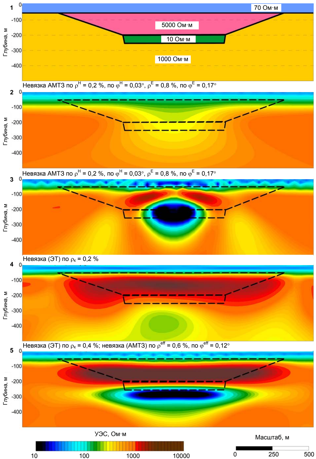
Рис.2. Синтетическая модель 2 высокоомной интрузии с проводником в основании
