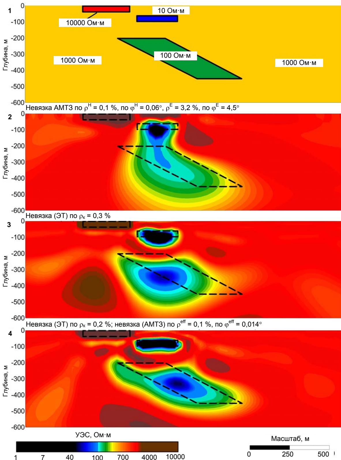
Рис.3. Синтетическая модель 3 наклонного проводника с приповерхностными неоднородностями
