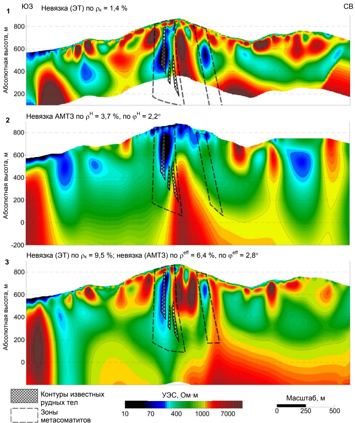
Рис.6. Месторождение Сигнальное
